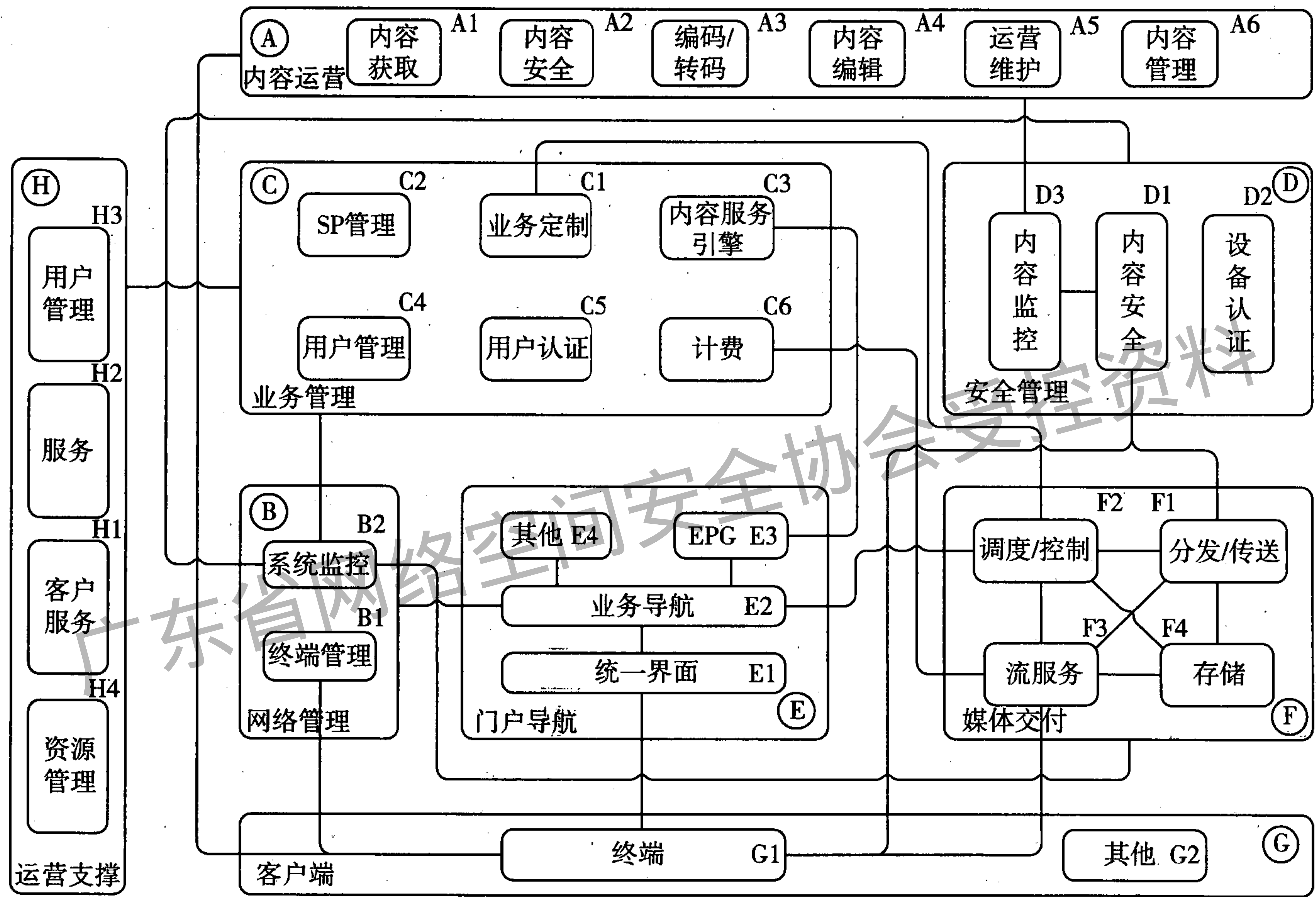
图 1 总体系架构图
