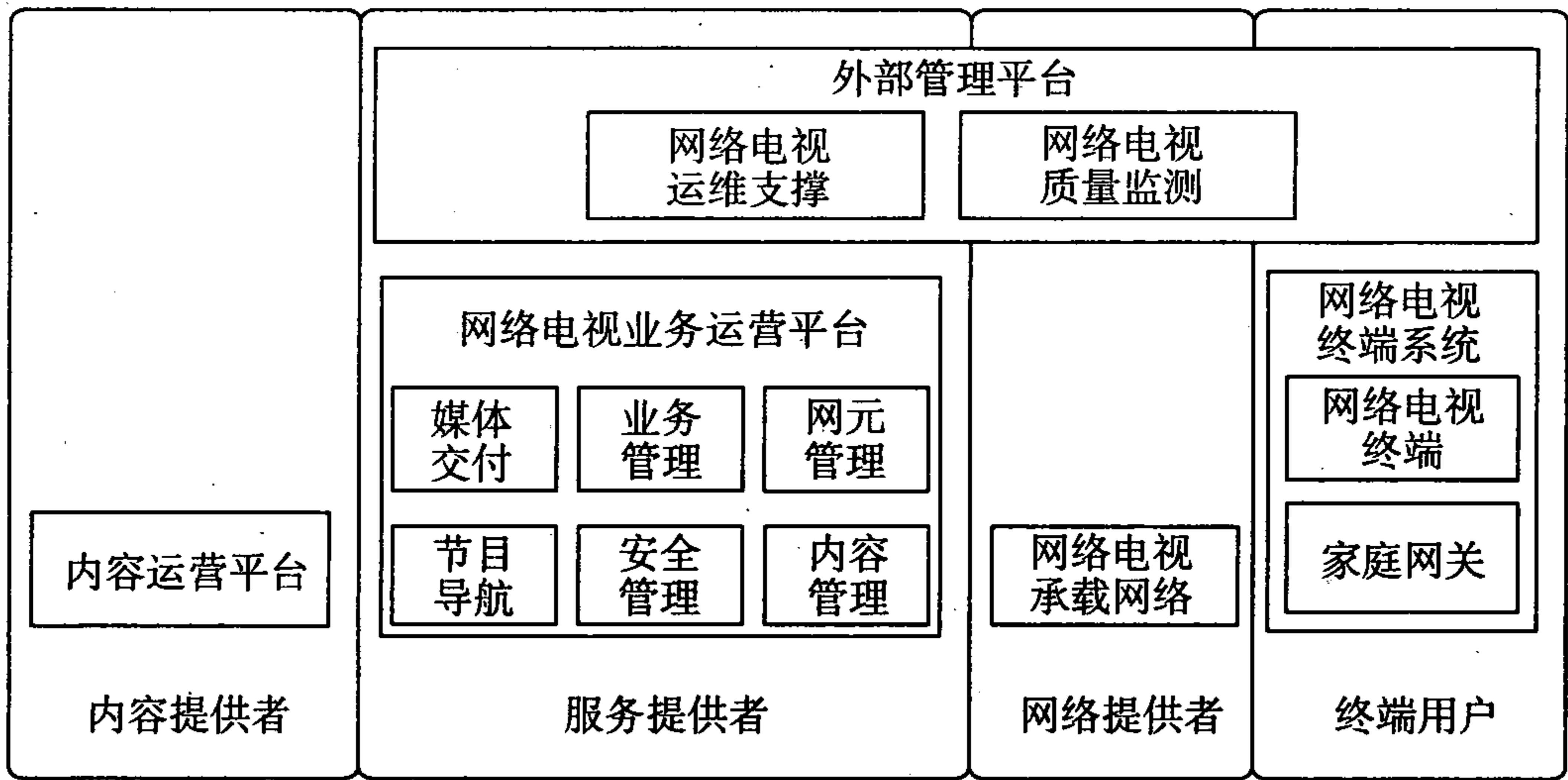
图 3.2.2 网络电视系统物理模型架构图
