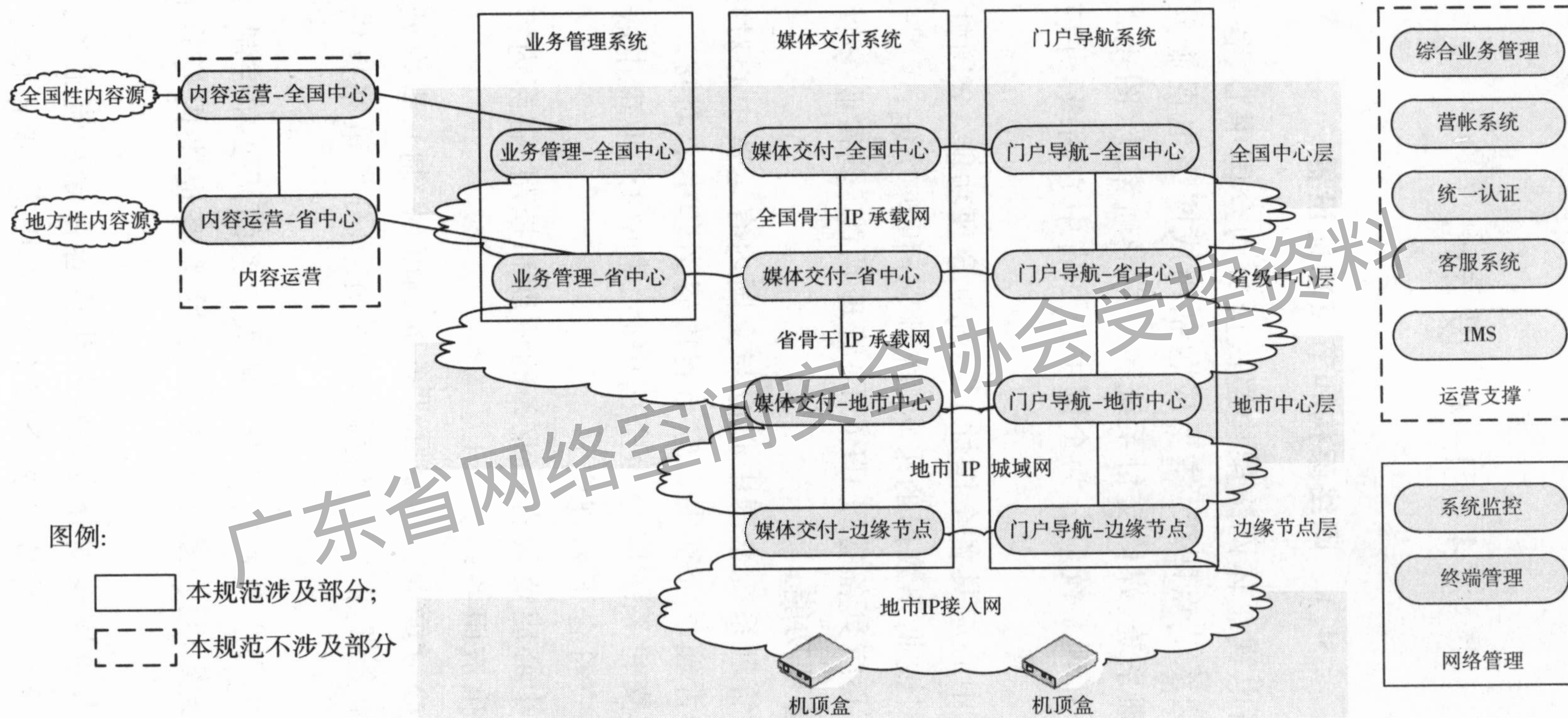
图 4.1.1 网络电视总体网络架构图
