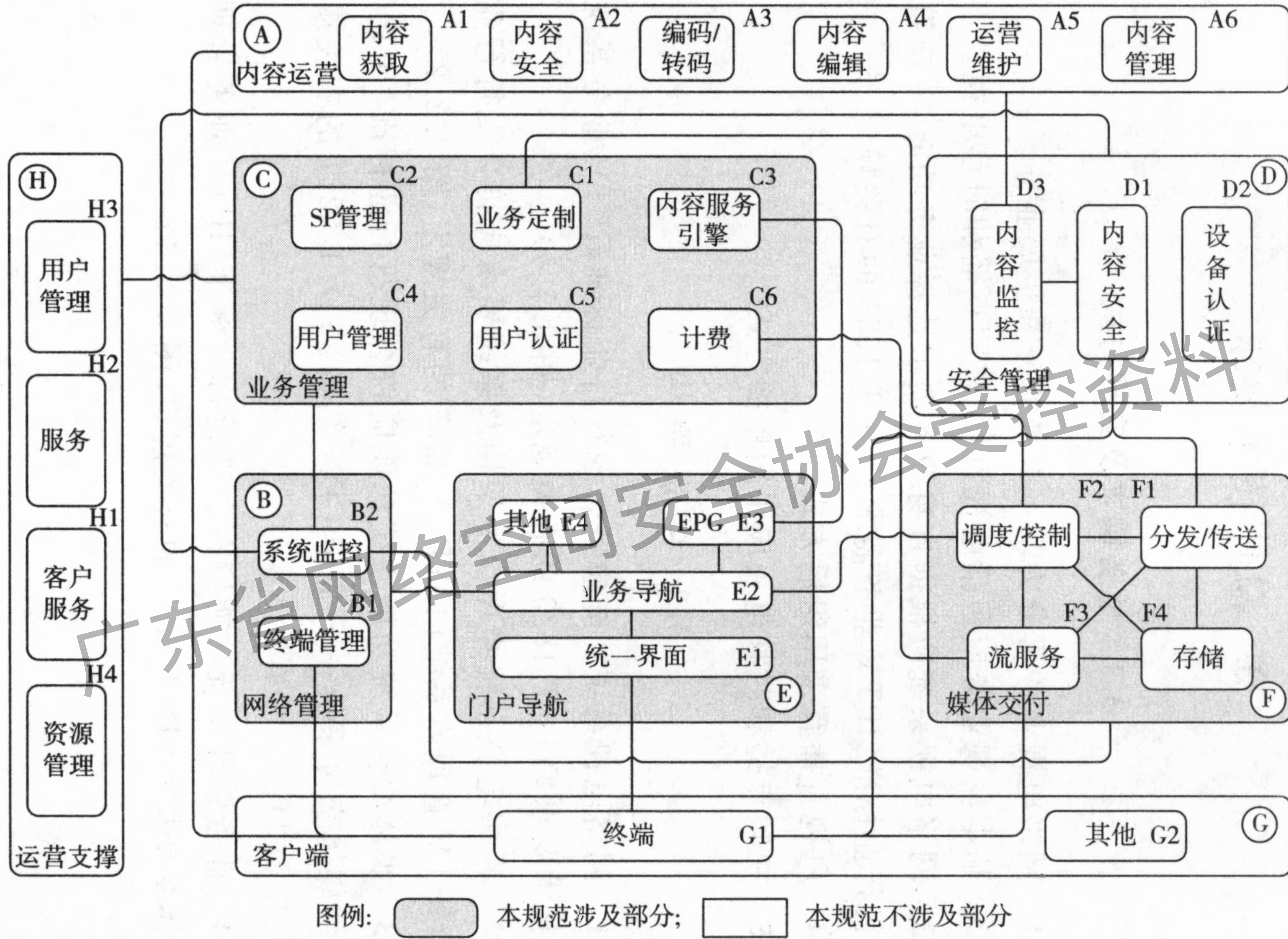
图 3.2.1 网络电视系统功能模型结构及接口图
