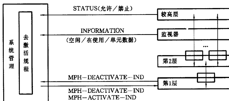
图 H1 去激活过程相互作用的概念模型举例
