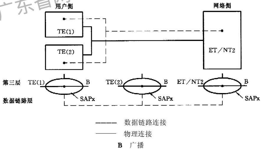
图 7 广播式数据链路连接
