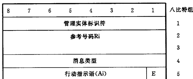
图 23 用于 TEI 管理程序的消息 在特定的消息中,不用的字段编码为全“0”,并且不由任一侧处理。 表 10 规定了各种消息中每个字段的编码。
