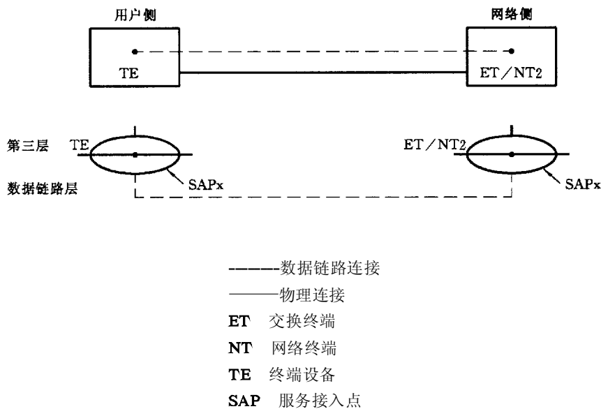
图 6 点到点数据链路连接
