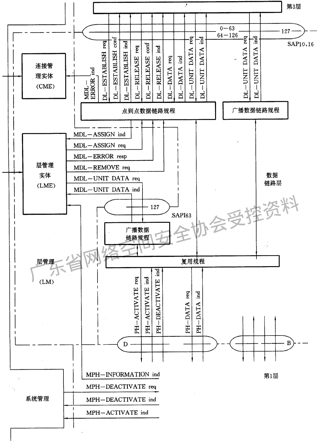
图 19 功能模块相互作用图
