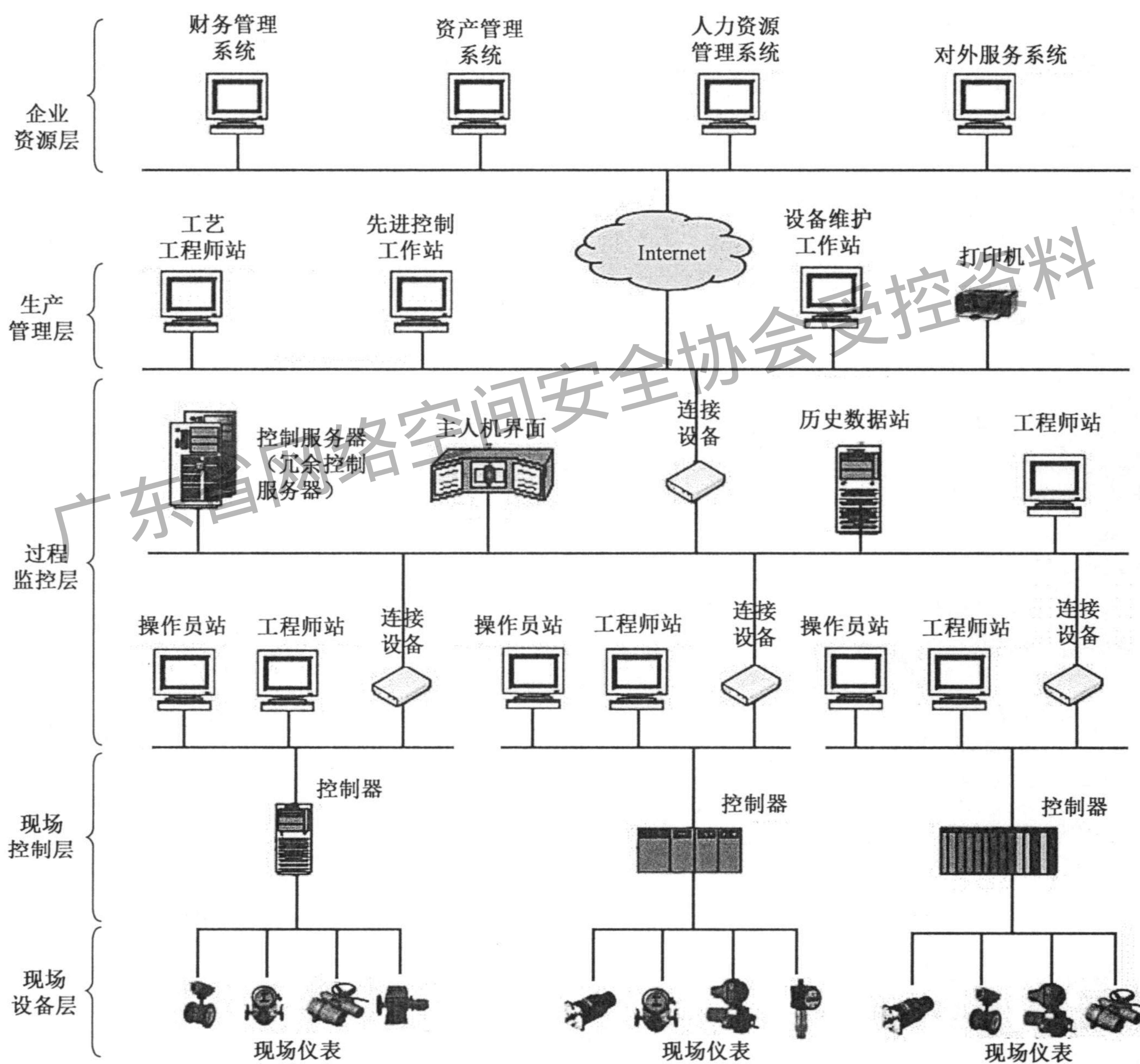
图 1 典型 DCS 系统的网络结构示意图
