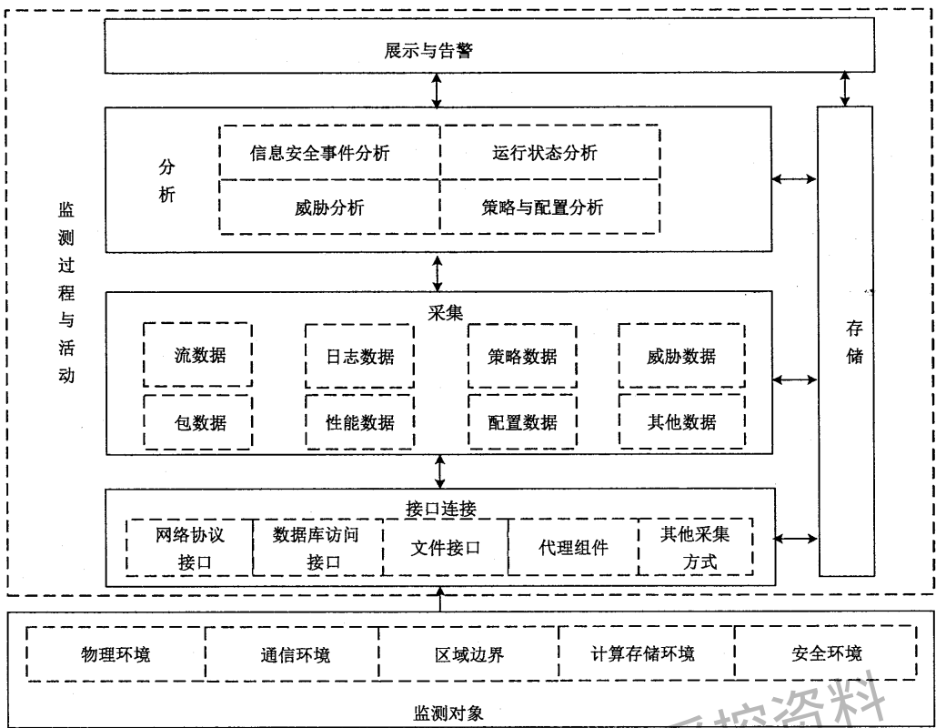
图 1 网络安全监测框架
