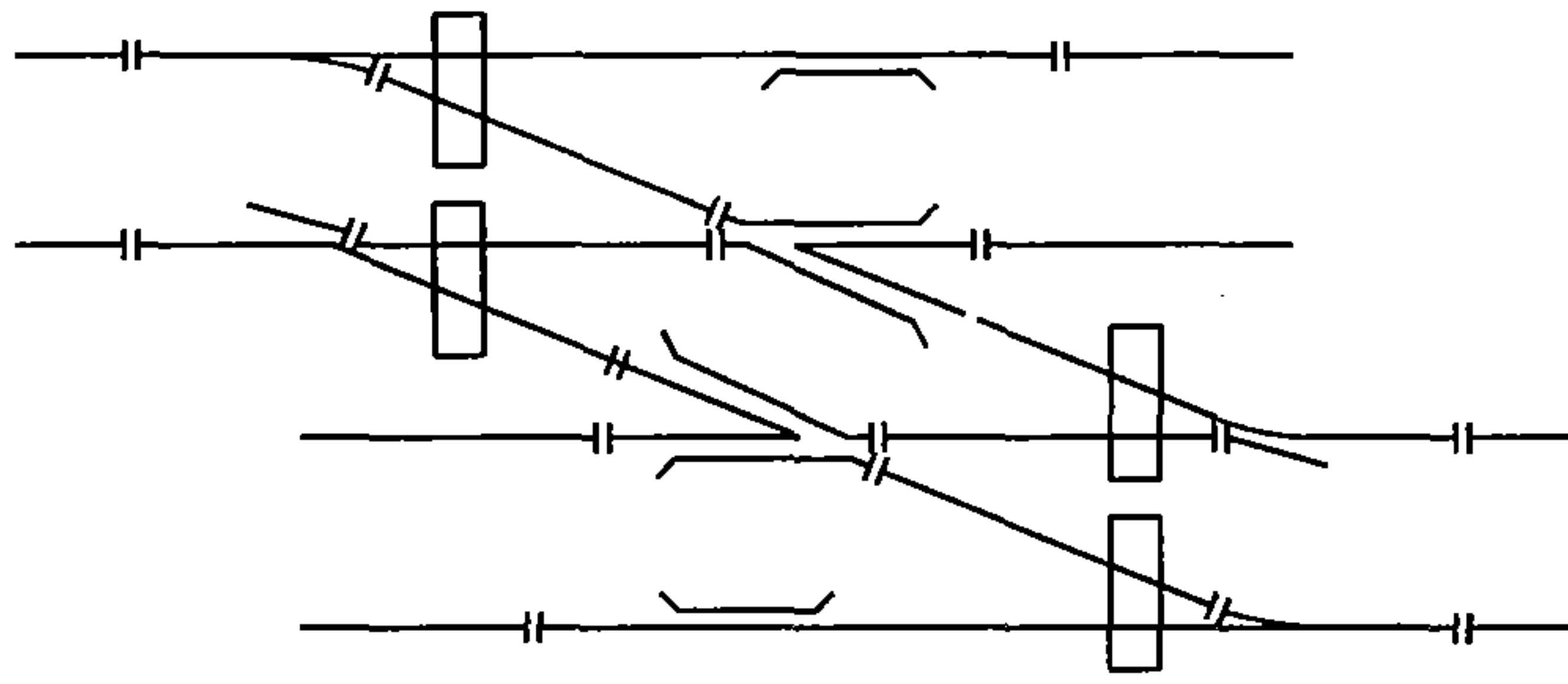
图 D3 渡线道岔连接图
