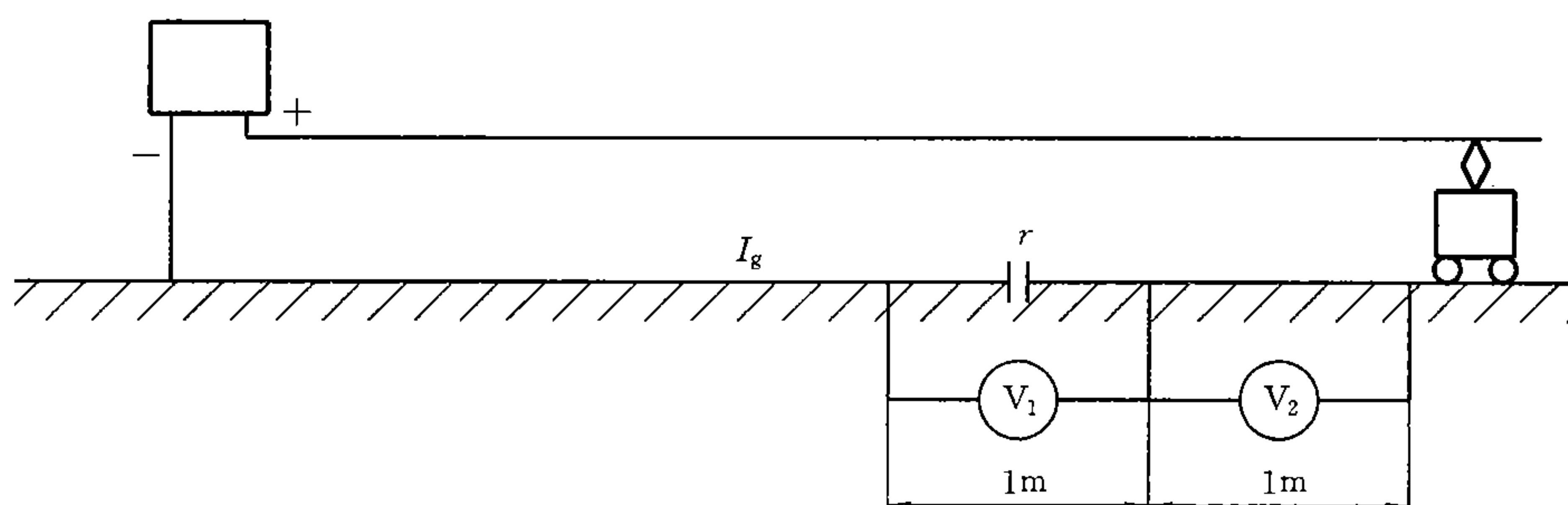
图 C1 测量轨道接缝电阻的接线方法
