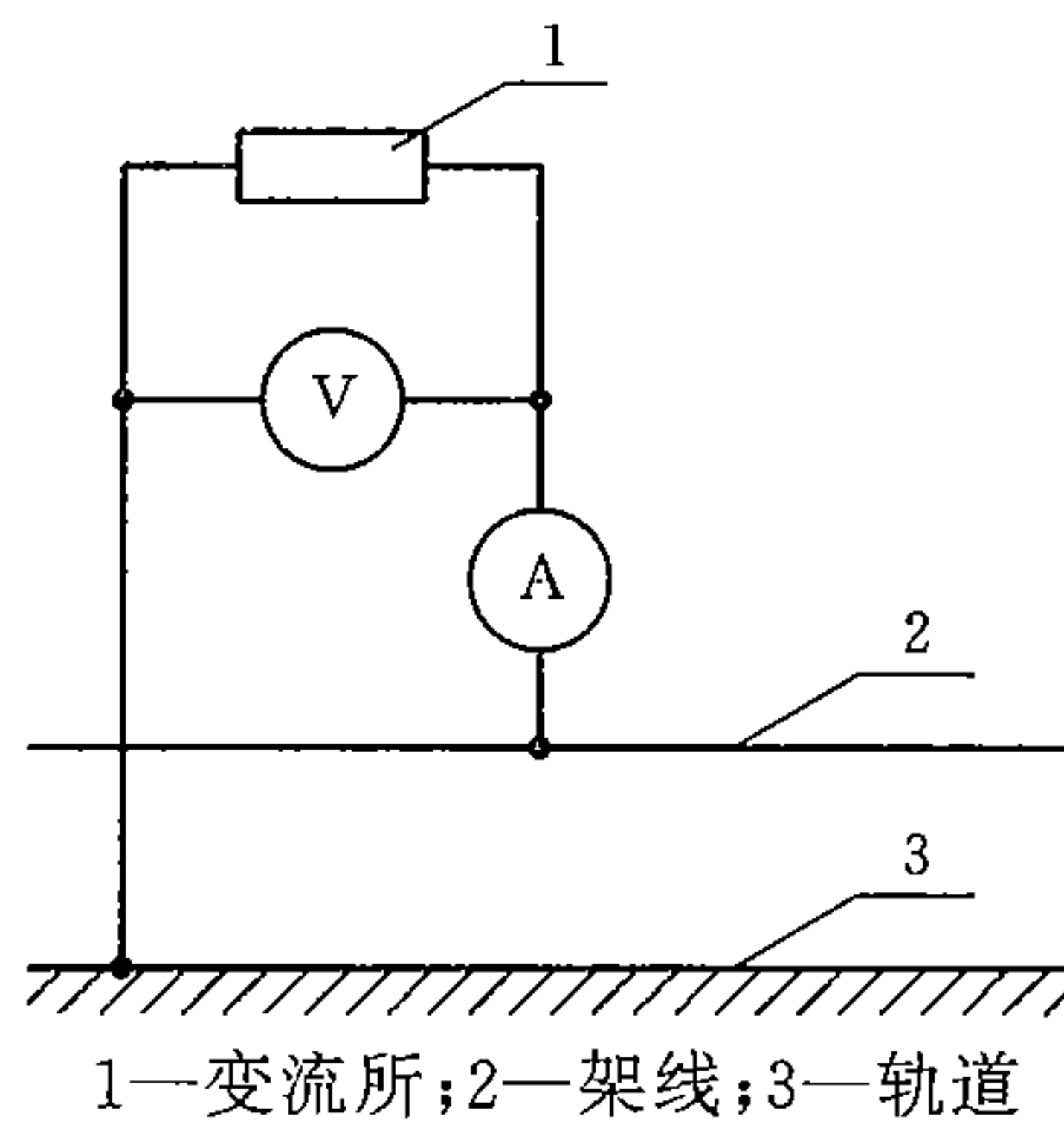
图 B1 测量漏泄电流的接线方法
