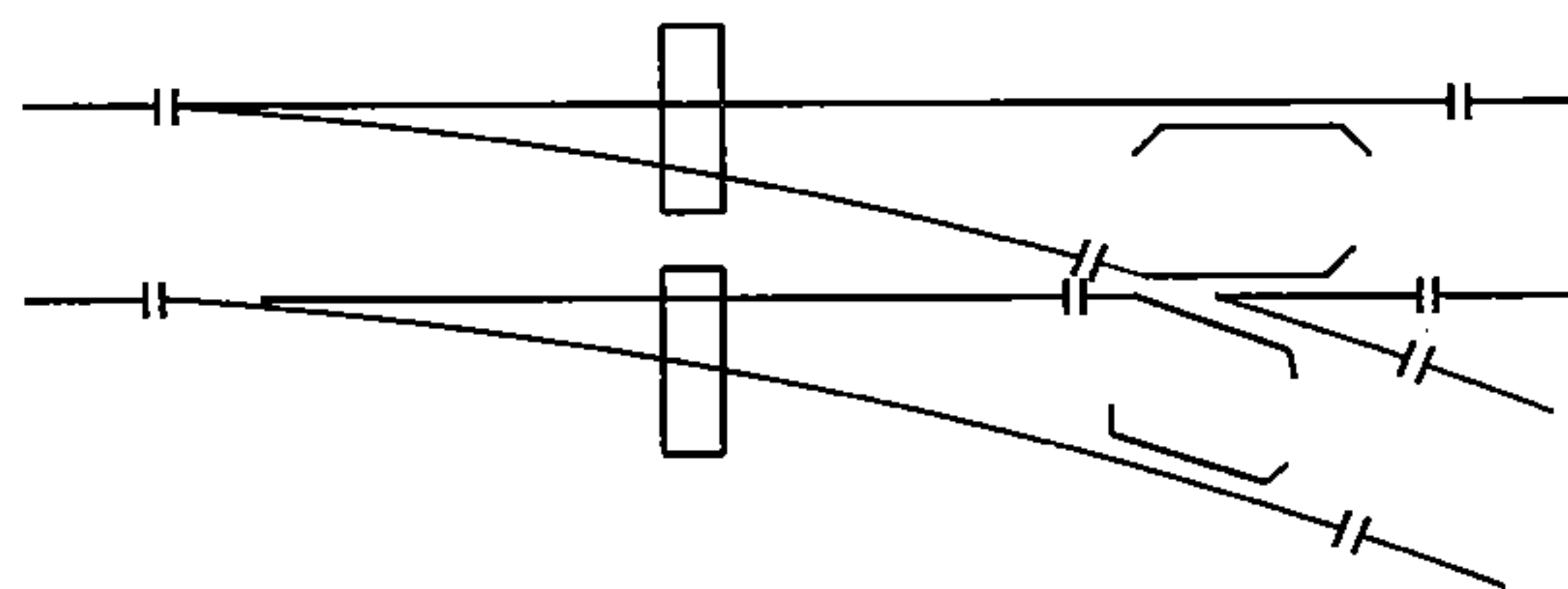
图 D1 单开道岔连接图
