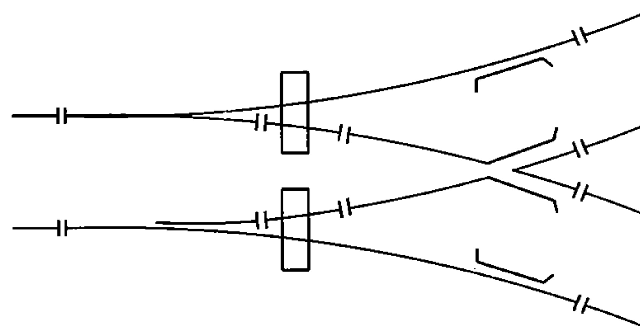
图 D2 对称道岔连接图
