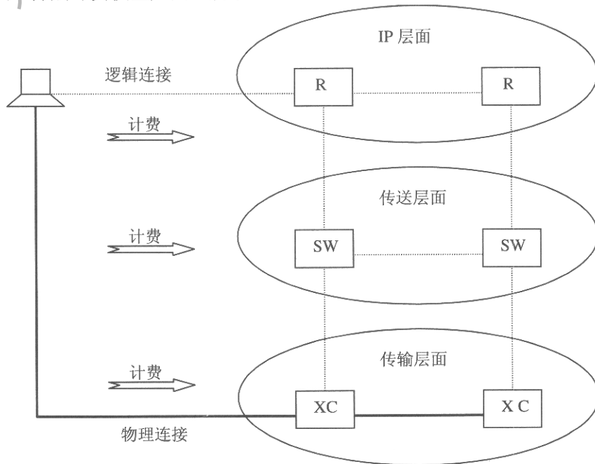
图 2 IP 网络分层计费模型
