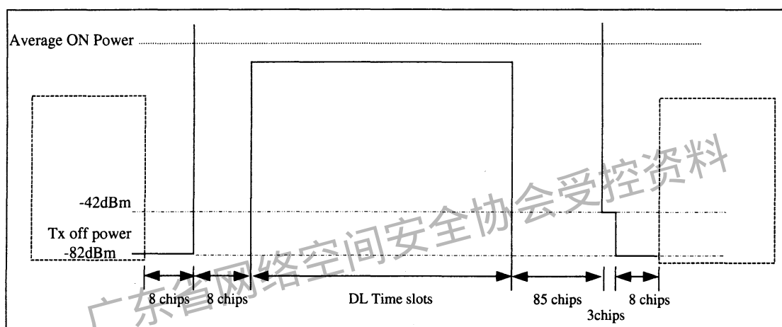
图 2 发射机开启 / 关闭时域模板
