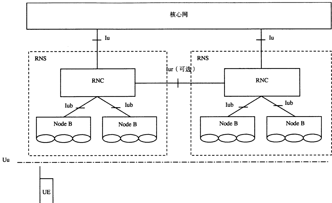
图 1 TD-SCDMA 无线网络网络 (RNS)
