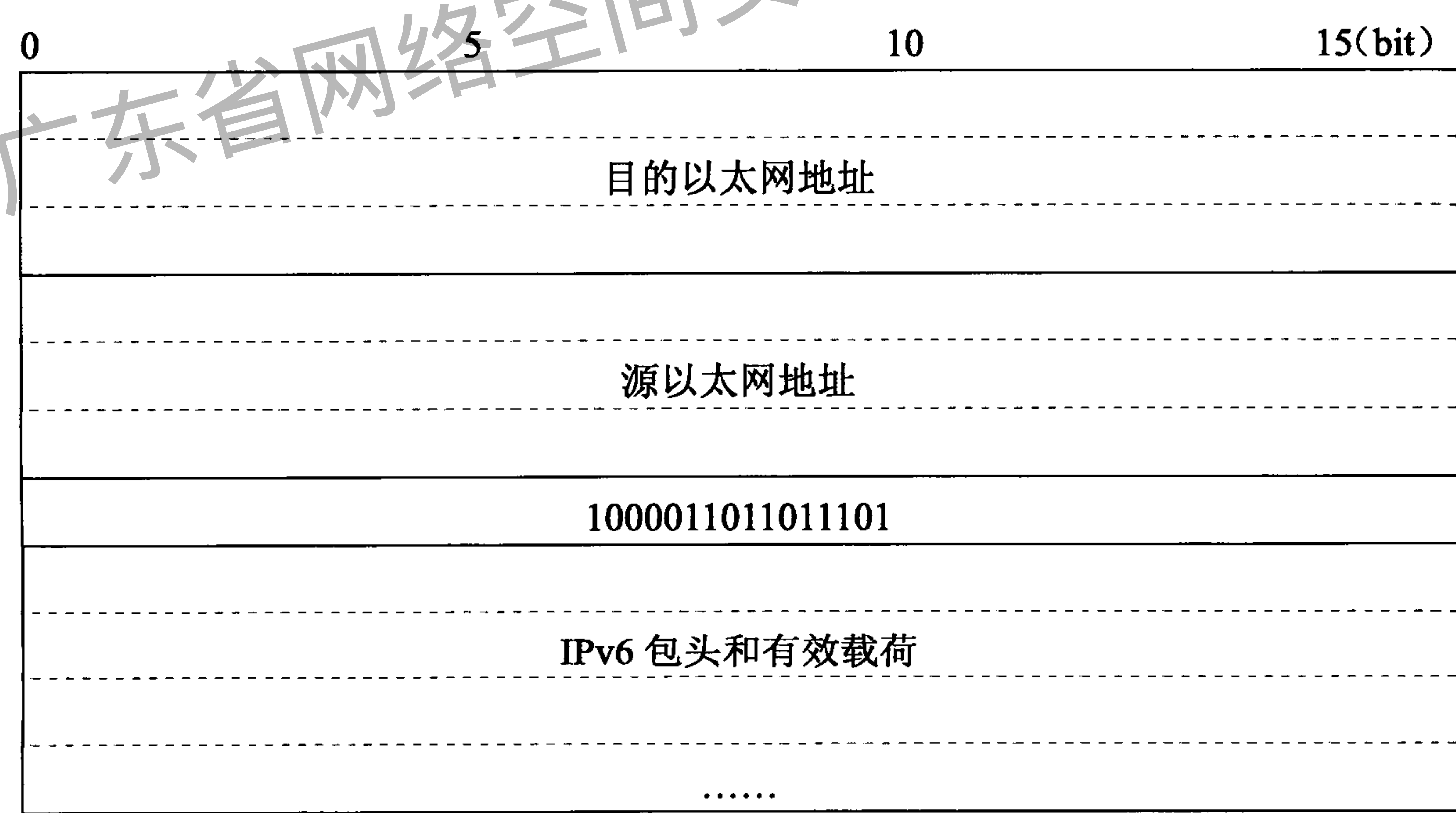
图 B.1 帧格式
