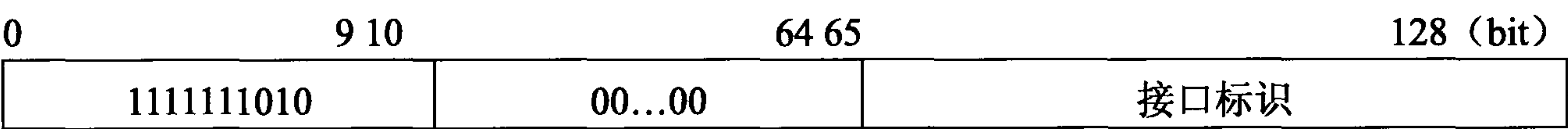
图 B.2 以太网接口的 IPv6 链路本地地址
