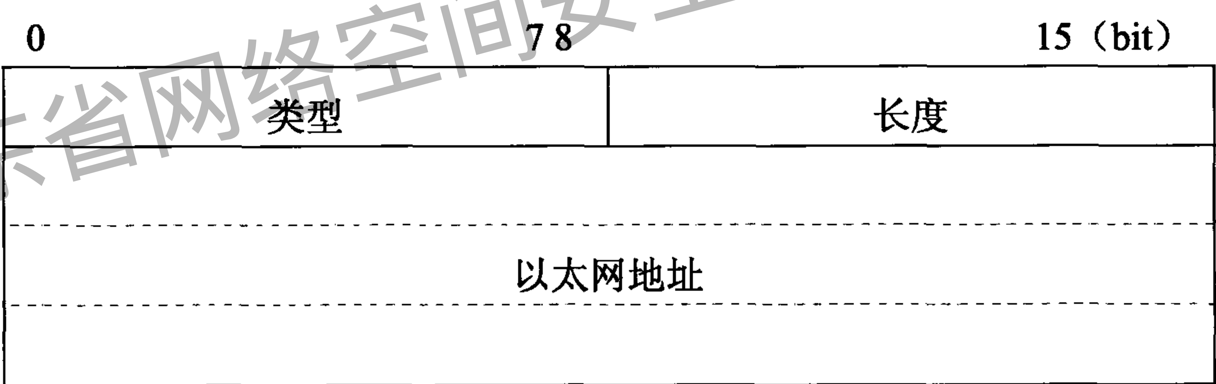
图 B.3 源/目的链路层地址选项格式
