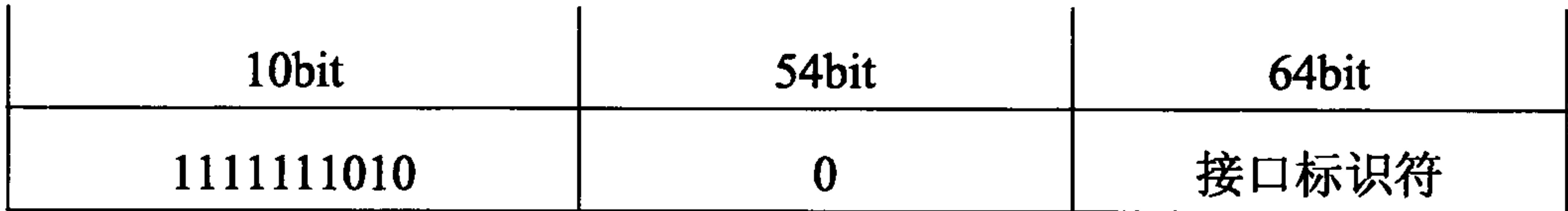
图 A.7 PPP 接口的链路本地地址格式
