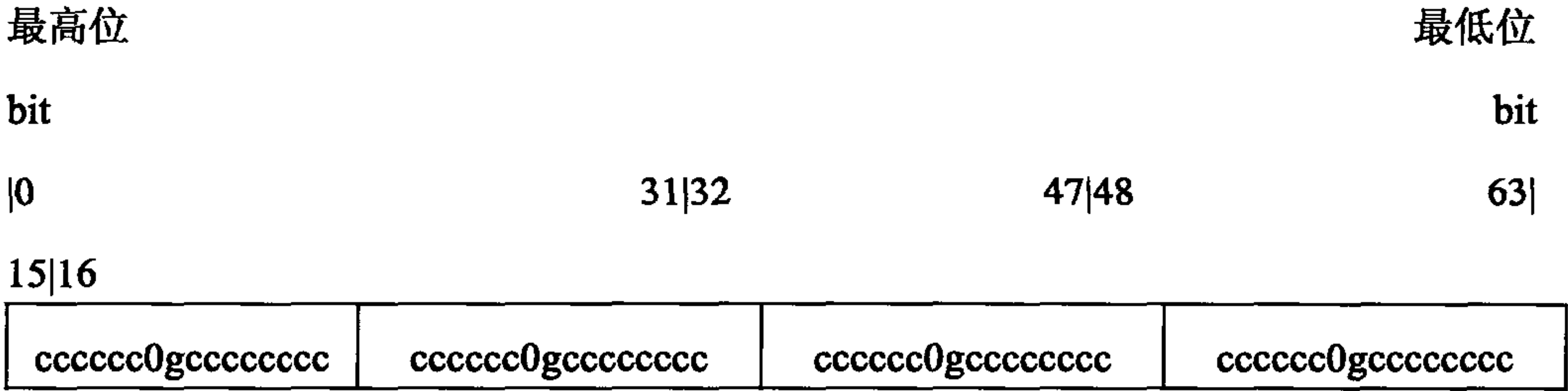
图 A.1 全球惟一的 EUI-64 标识符格式
