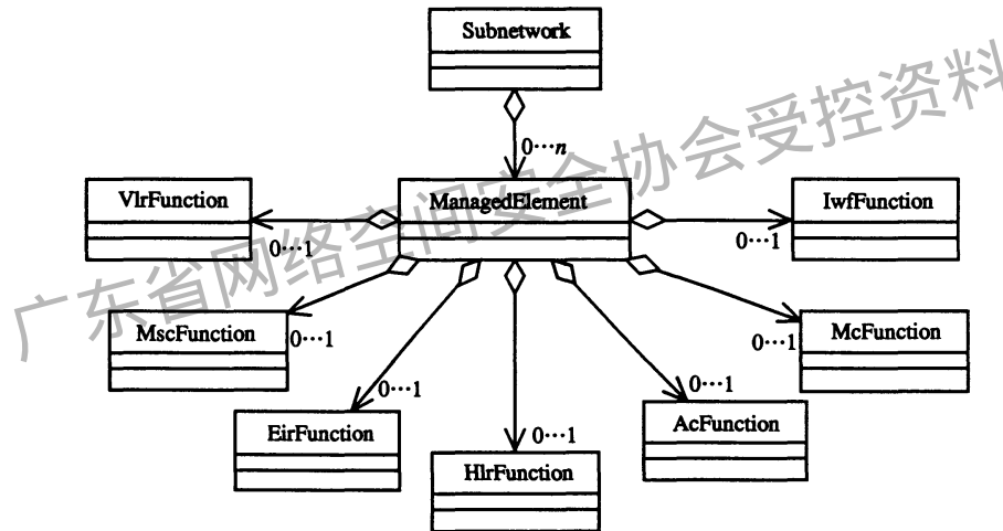
图6 核心网电路域配置网络资源对象包含关系图 (1)
