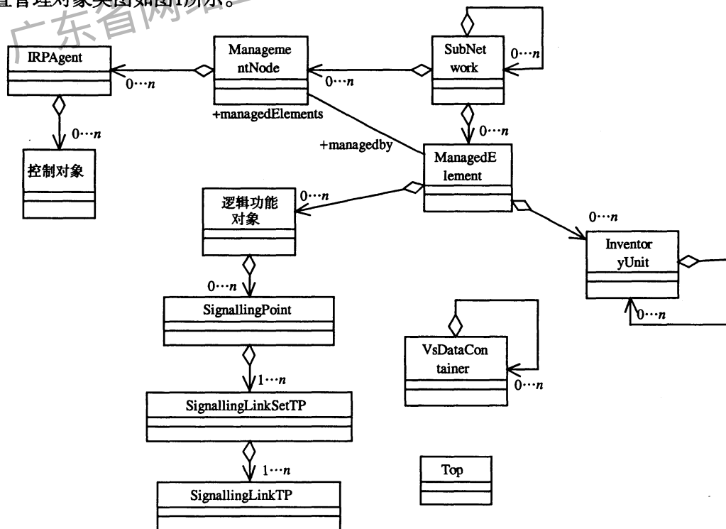
图1 通用配置网络资源模型包含关系 1
