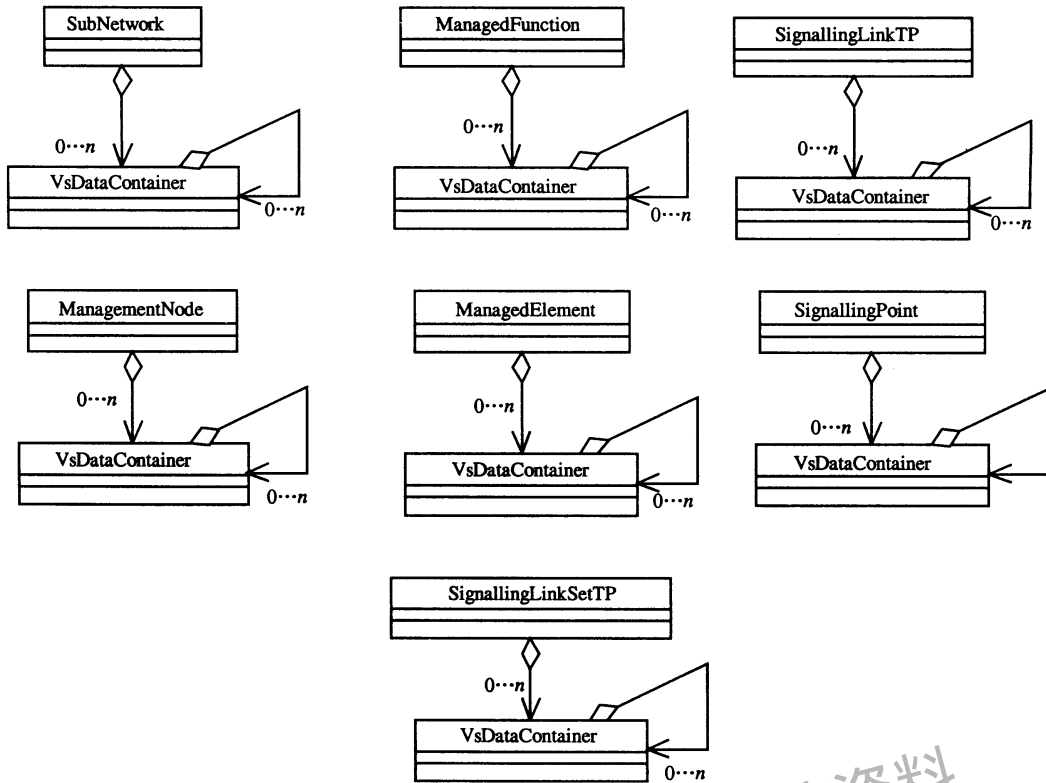
图2 通用配置网络资源模型包含关系 2
