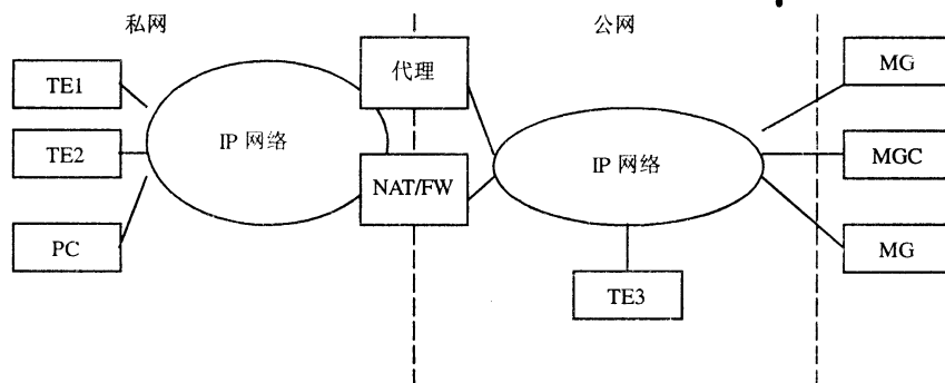
图3 MGCP代理处于一级公私网边缘
