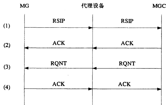
图7 代理处于私网通信流程——转发单端点注册流程
