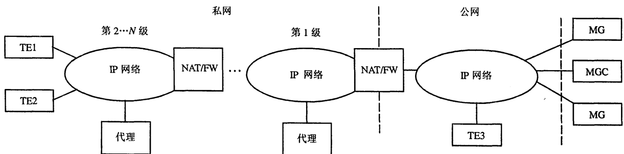
图2 MGCP代理处于多级私网
