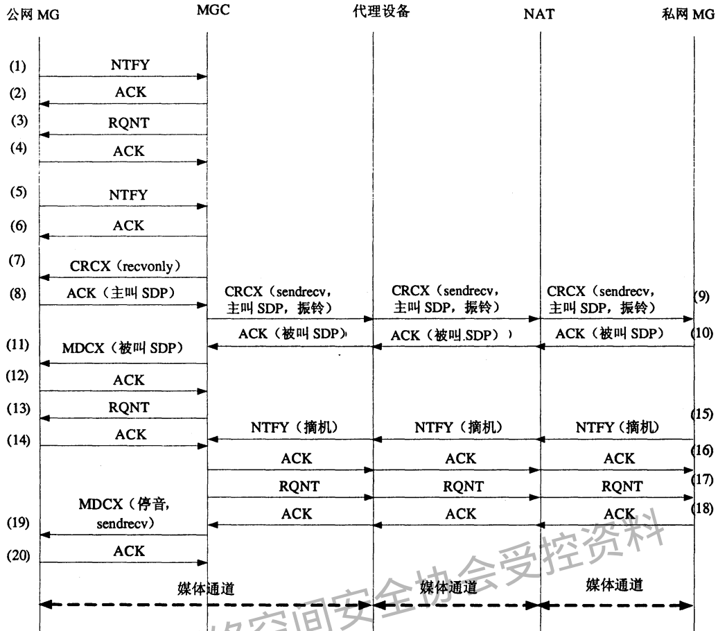
图17 代理处于公网的通信流程——公网到私网的呼叫流程
