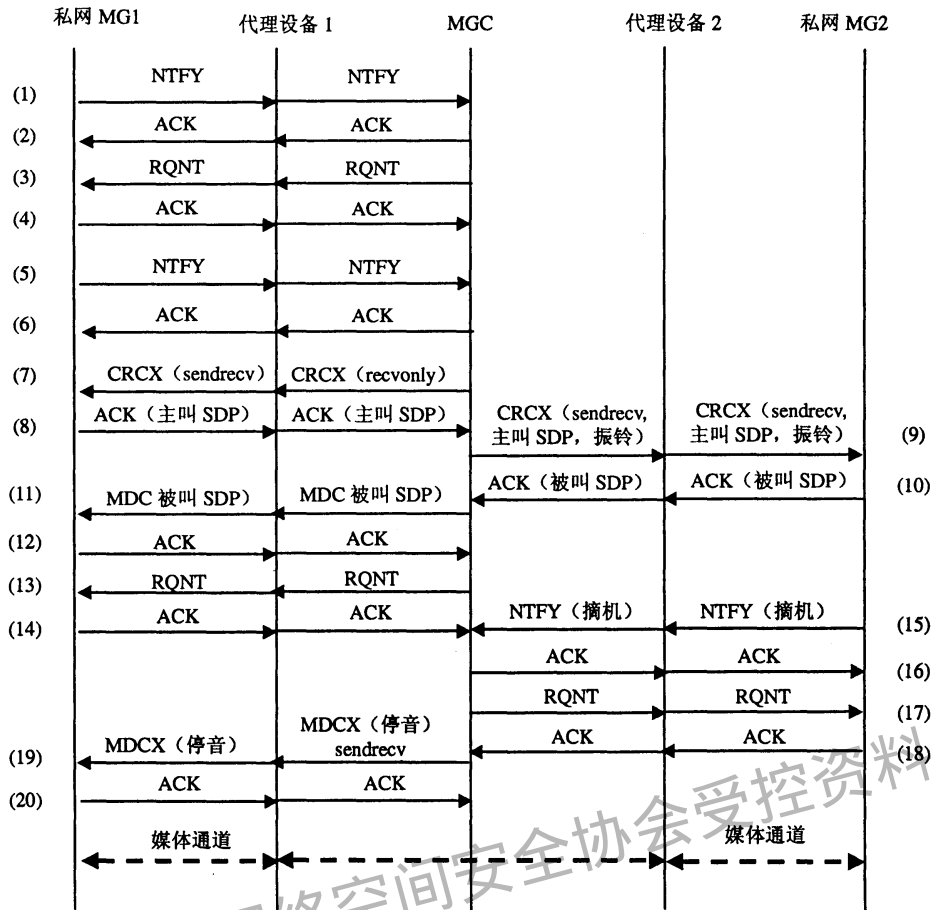
图11 代理处于私网通信流程——私网终端呼叫属于同一 MGC（不同代理设备）的私网终端
