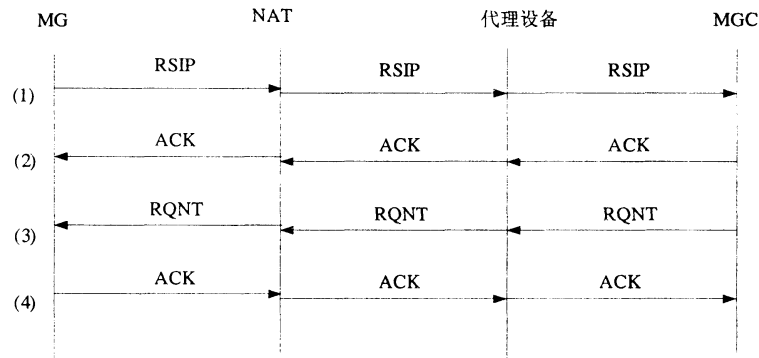
图14 代理处于公网的通信流程——转发单端点注册流程
