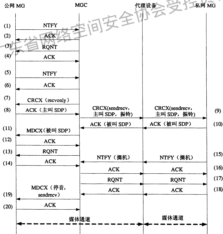
图10 代理处于私网通信流程——公网向私网发起呼叫
