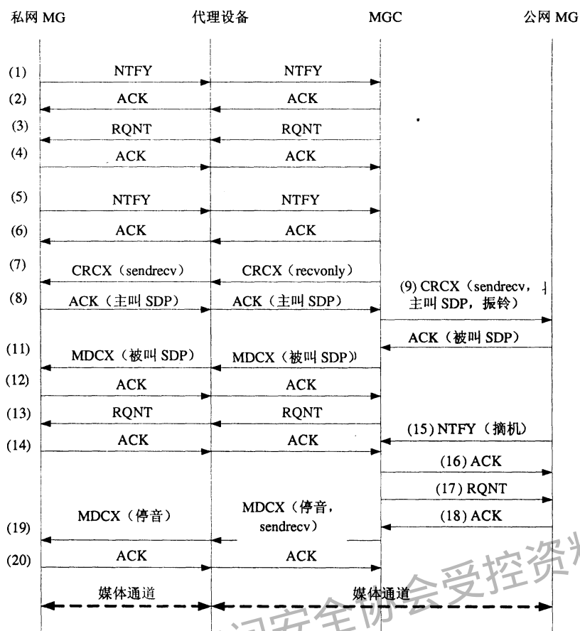
图9 代理处于私网通信流程——私网向公网发起呼叫
