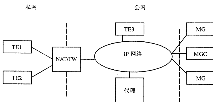
图5 MGCP代理处于公网
