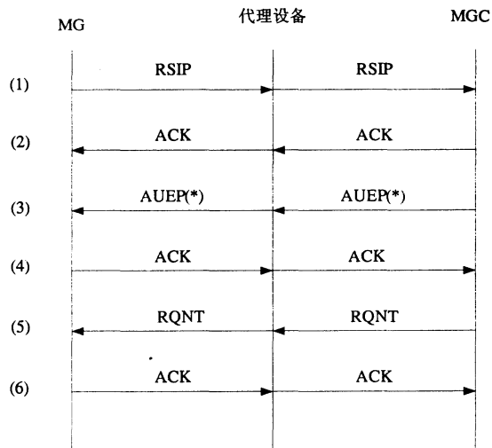
图6 代理处于私网通信流程——转发开机注册流程
