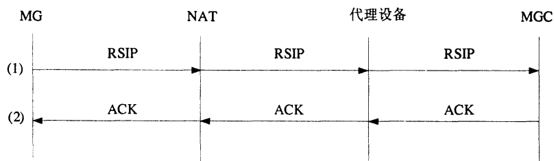
图15 代理处于公网的通信流程——注销流程
