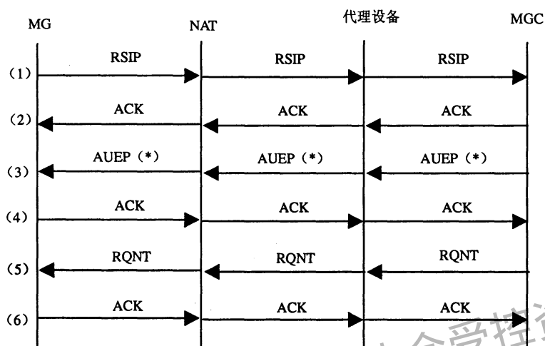
图13 代理处于公网的通信流程——转发开机注册流程
