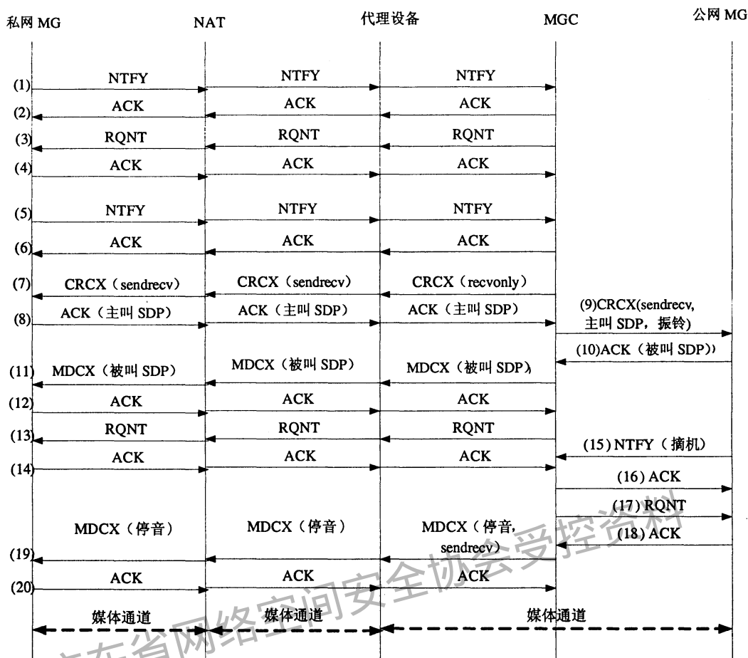
图16 代理处于公网的通信流程——私网到公网的呼叫流程
