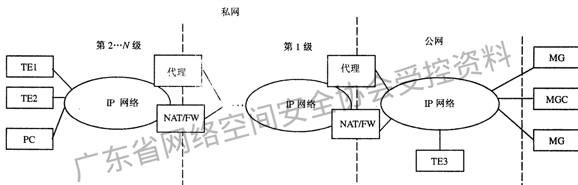
图4 MGCP代理处于多级公私网络边缘
