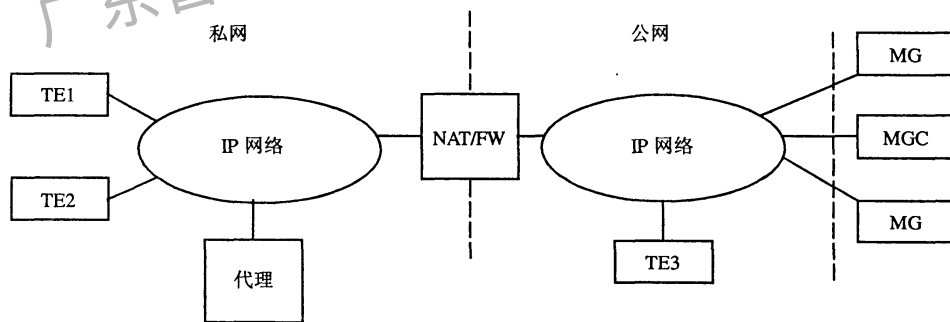
图1 MGCP代理处于一级私网
