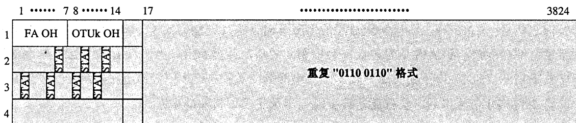
图25 ODUk-OCI
