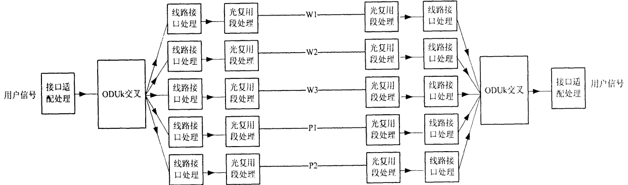
图47 不同光纤路径的 M:N ODUk SNCP
