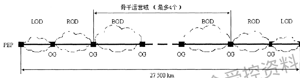
图38 假定参考光通道
