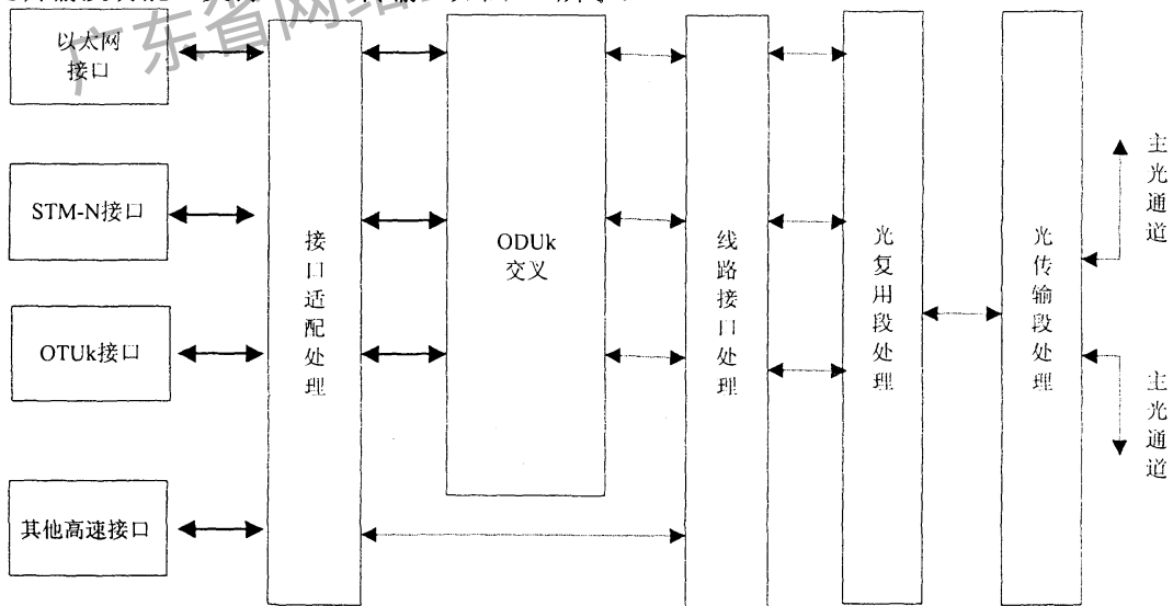
图44 OTN 电交叉设备的功能模型
