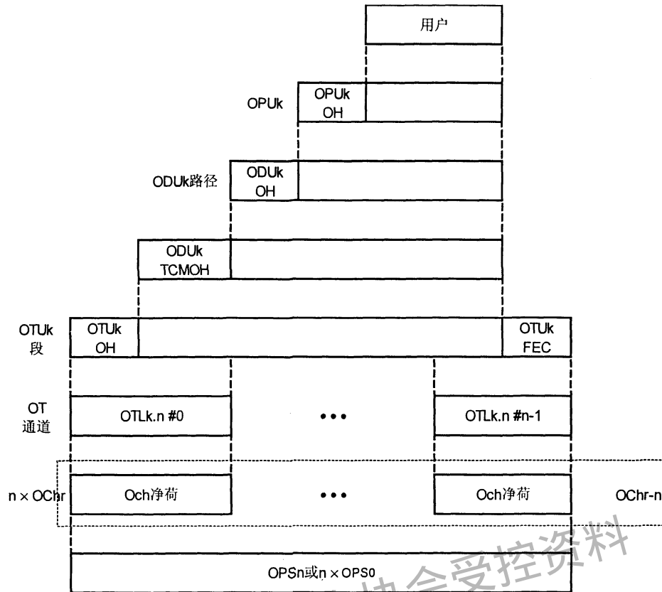
图12 OTM-0.myn 基本信息包含关系
