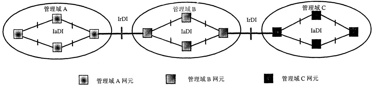
图8 OTN 网络分域
