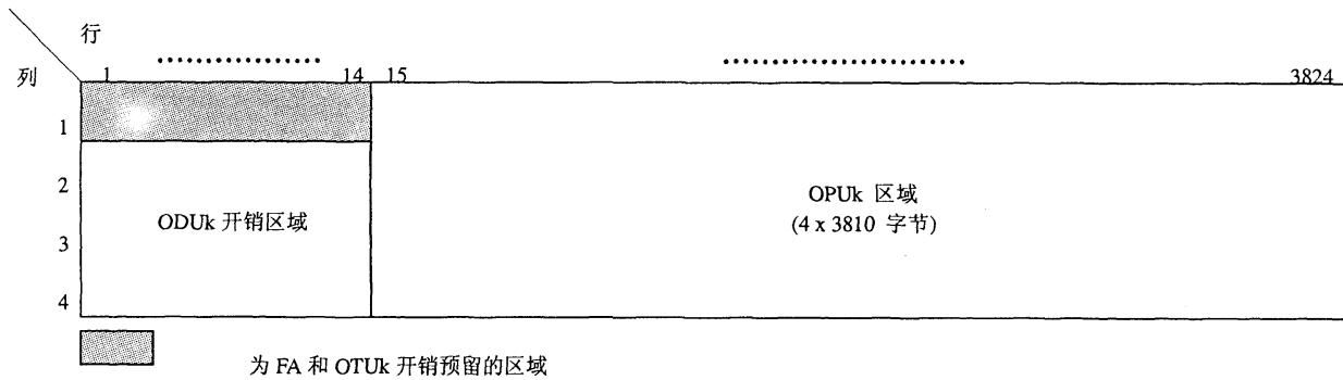
图18 ODUk 帧结构
