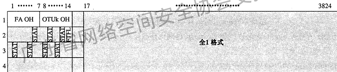
图24 ODUk-AIS
