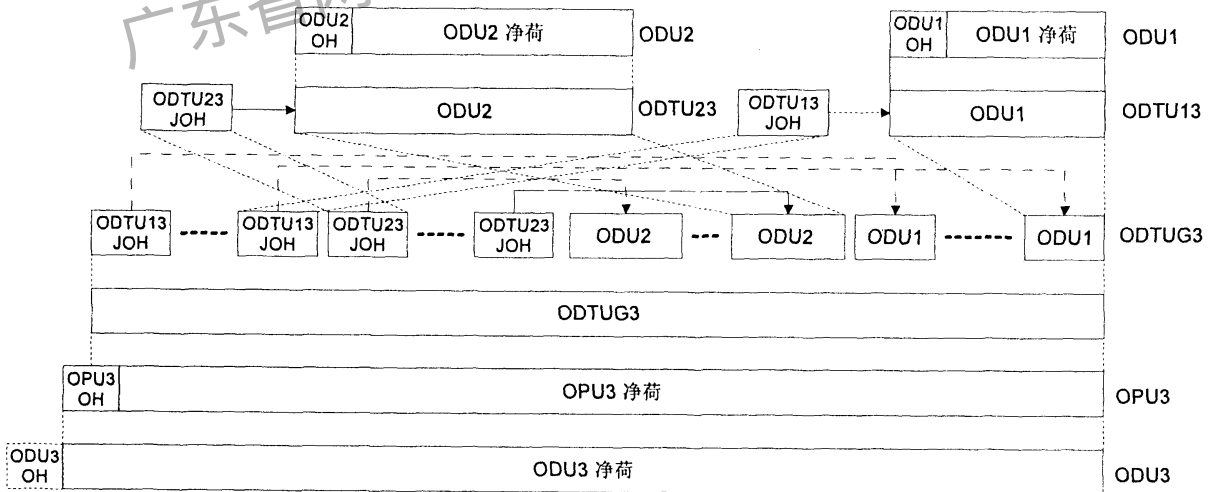
图31 ODU1 和 ODU2 复用到 ODU3
