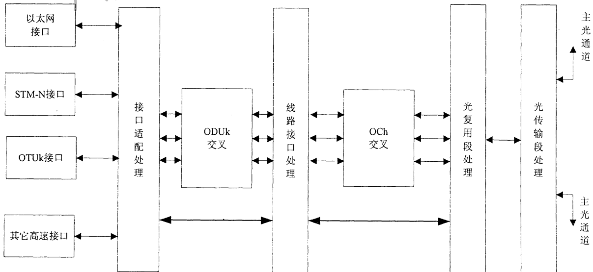
图45 OTN 光电混合交叉调度设备的功能模型
