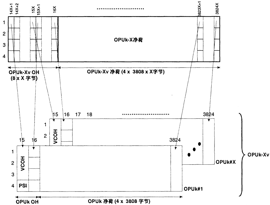
图36 OPUk-Xv 结构
