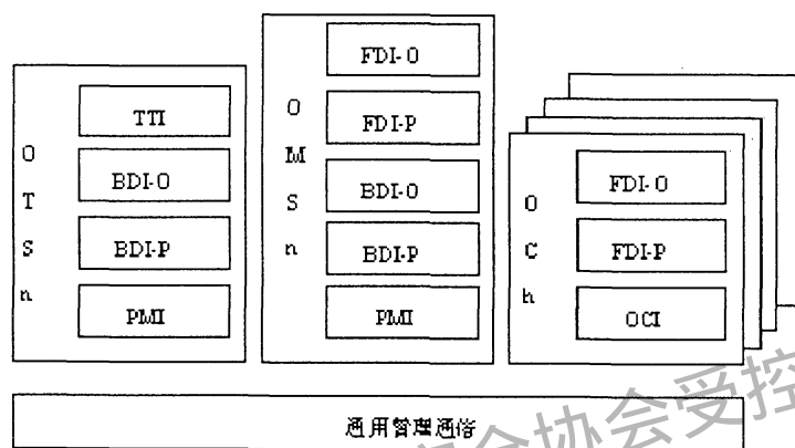
图22 OTSn, OMSn 和 OCh 开销作为 OOS 中的逻辑单元
