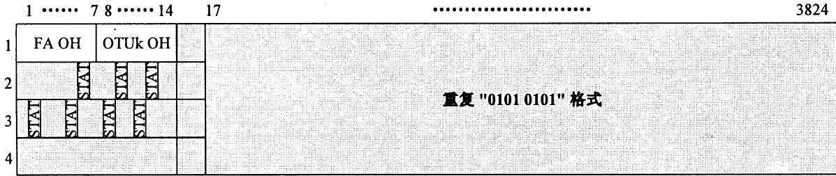
图26 ODUk-LCK
