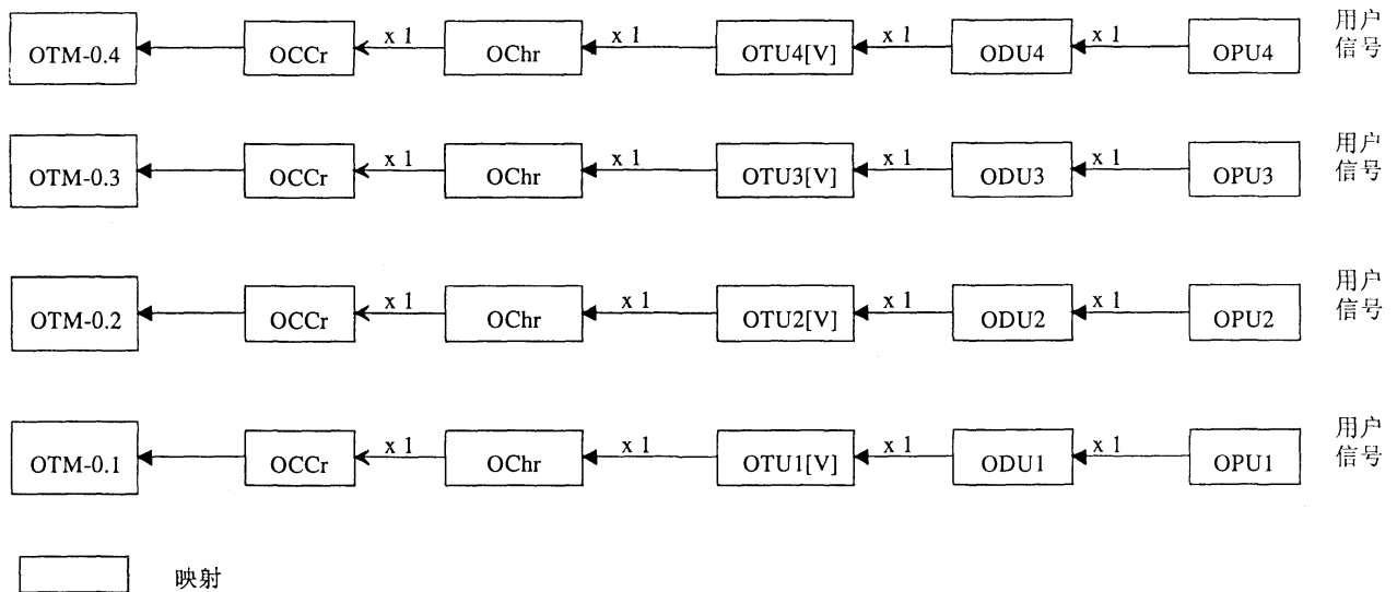
图33 OTM-0.m 结构
