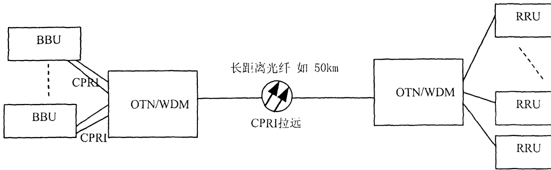
图 D.2 点到点或星型组网
