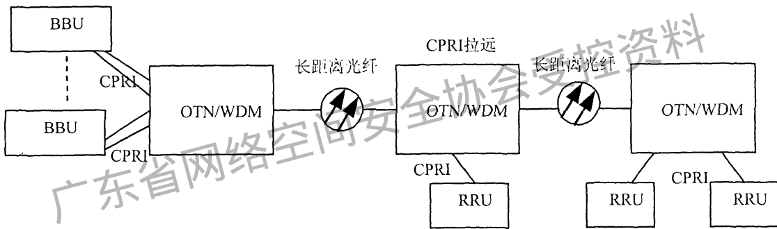
图 D.3 链型组网
