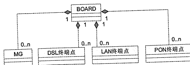
图9 设备信息模型
