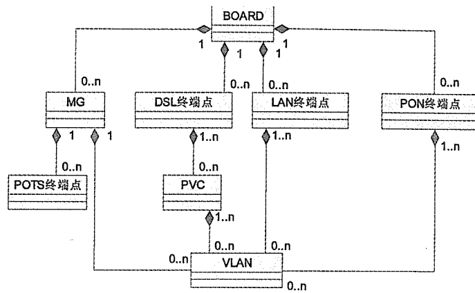
图11 终端点单元管理
