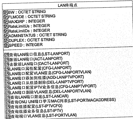
图14 LAN 终端点 UML 图
