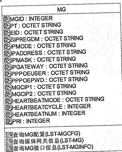
图17 媒体网关信息模型 UML 图
