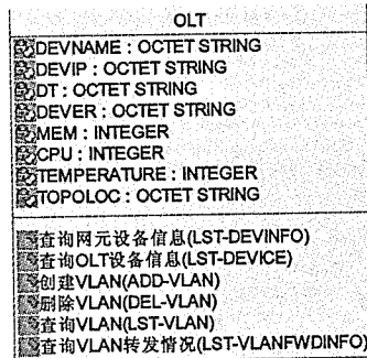
图5 网元 OLT 管理单元信息模型 UML 图
