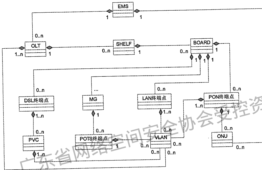
图1 通用对象管理
