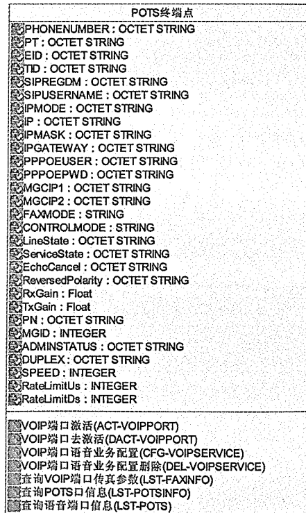
图13 POTS 终端点 UML 图
