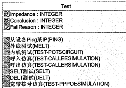
图19 测试诊断信息模型 UML 图
