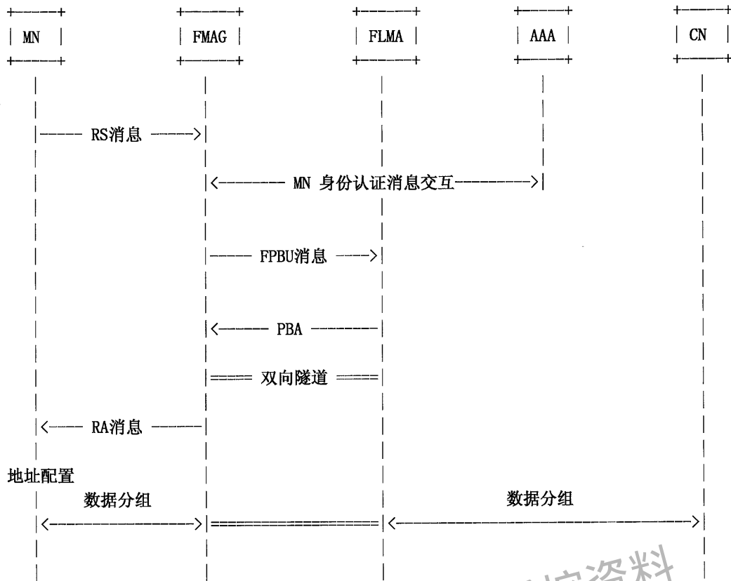
图7 初始化消息交互流程
