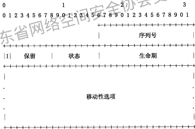
图4 FMA 消息报文格式
