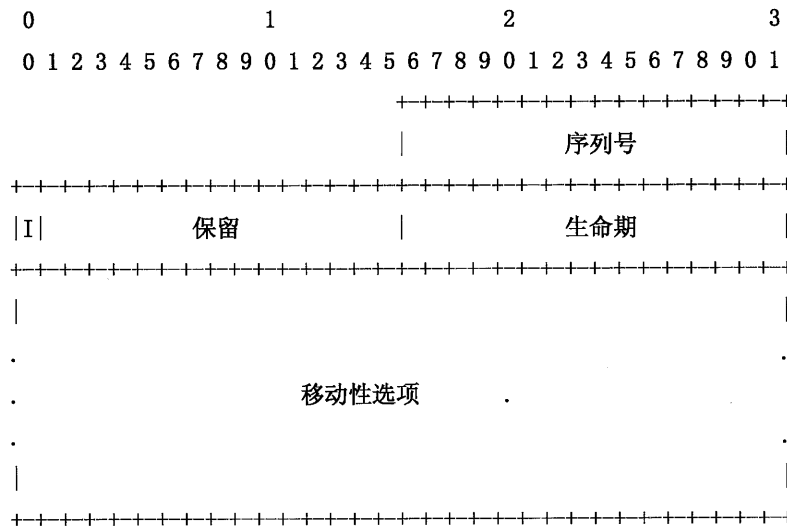
图3 FMI 消息报文格式
