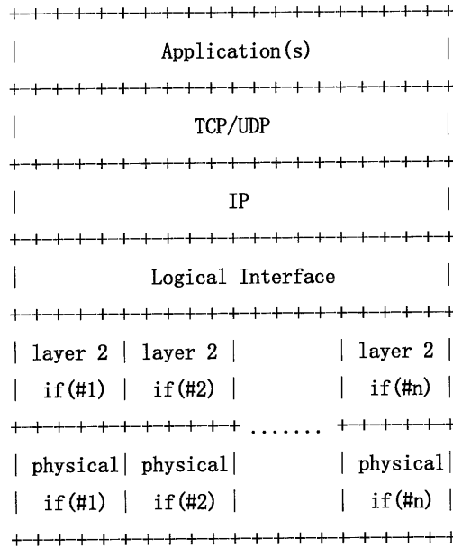
图2 逻辑接口在协议栈中的位置
