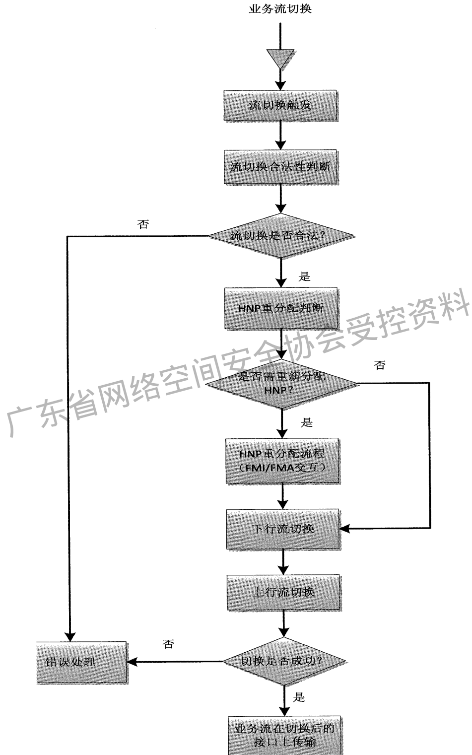
图8 业务流切换流程
