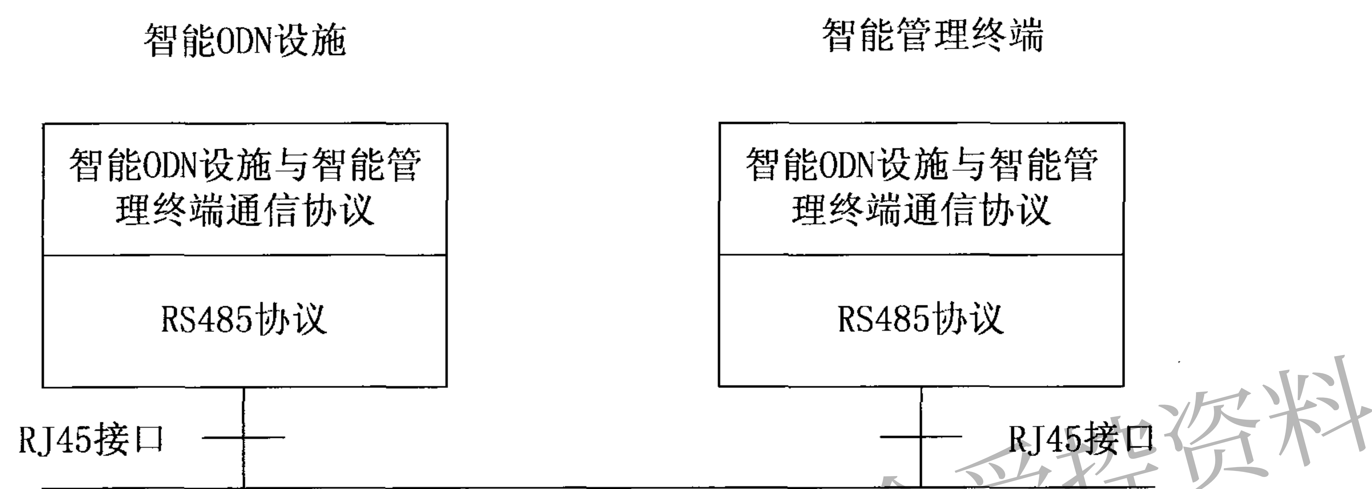
图2 I2 接口结构示意图
