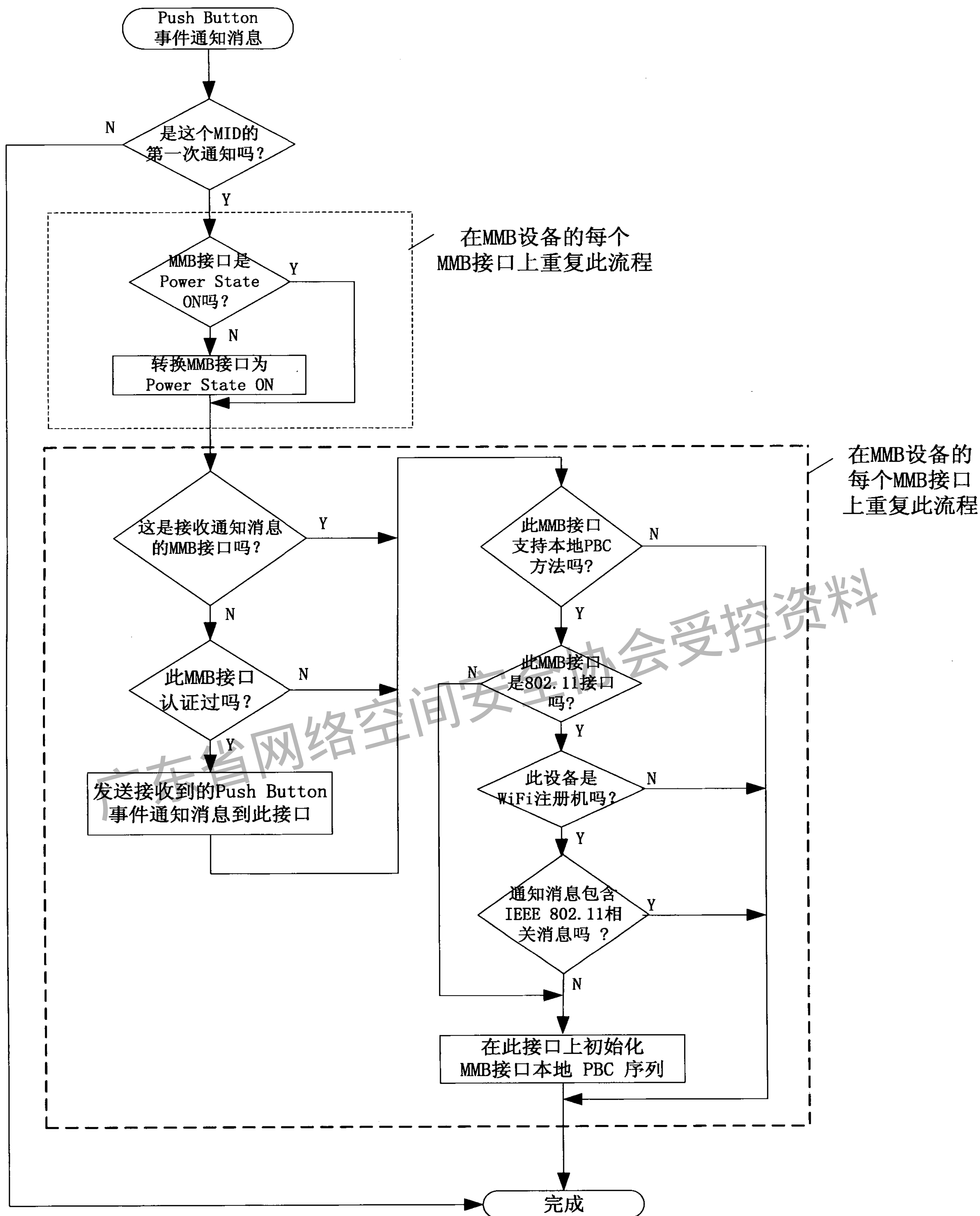
图5 Push Button 事件通知消息处理流程
