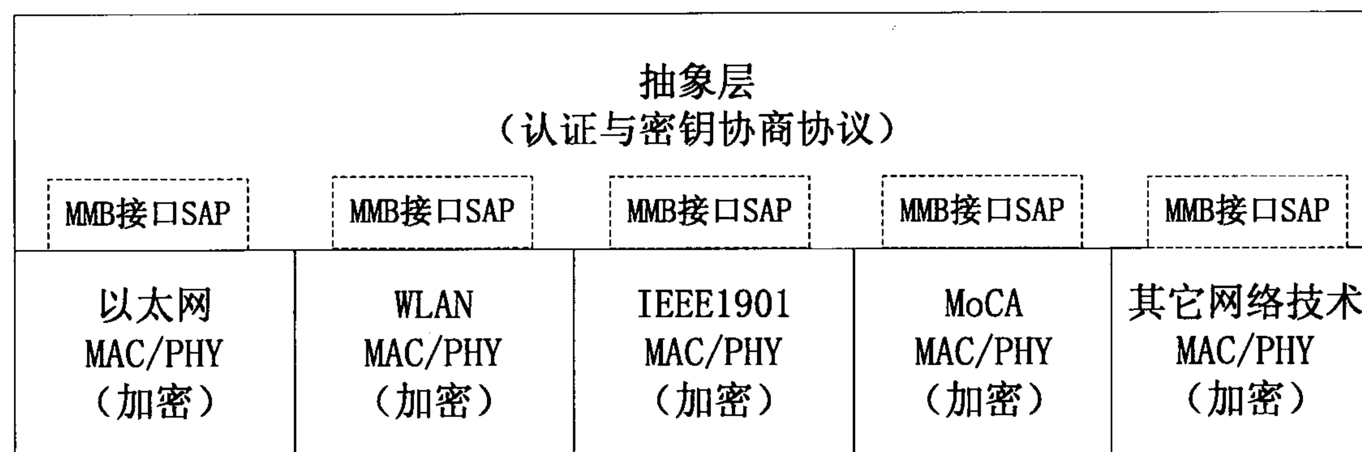
图3 MMB 安全建立架构
