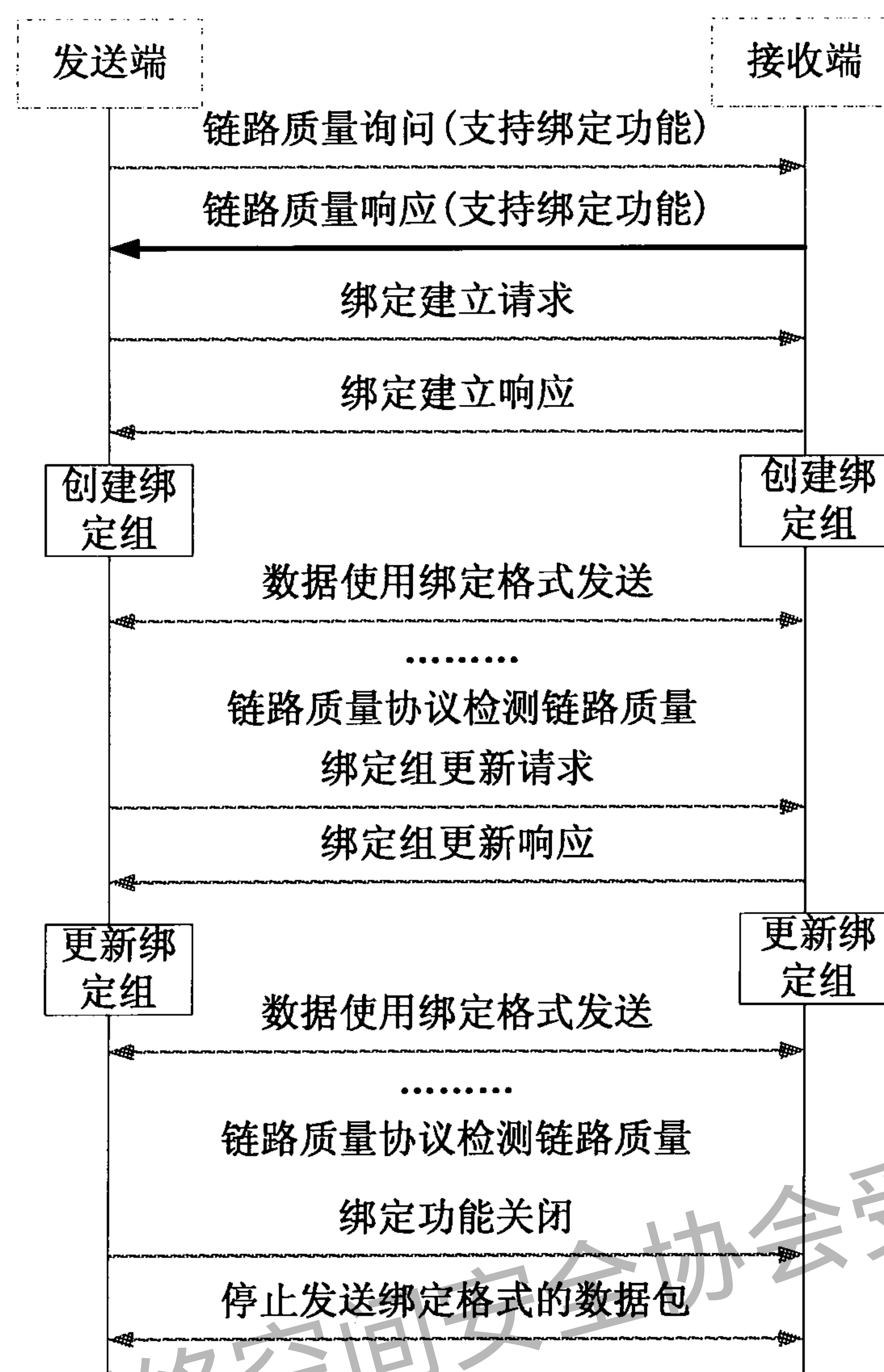
图11 多介质链路绑定协议流程图
