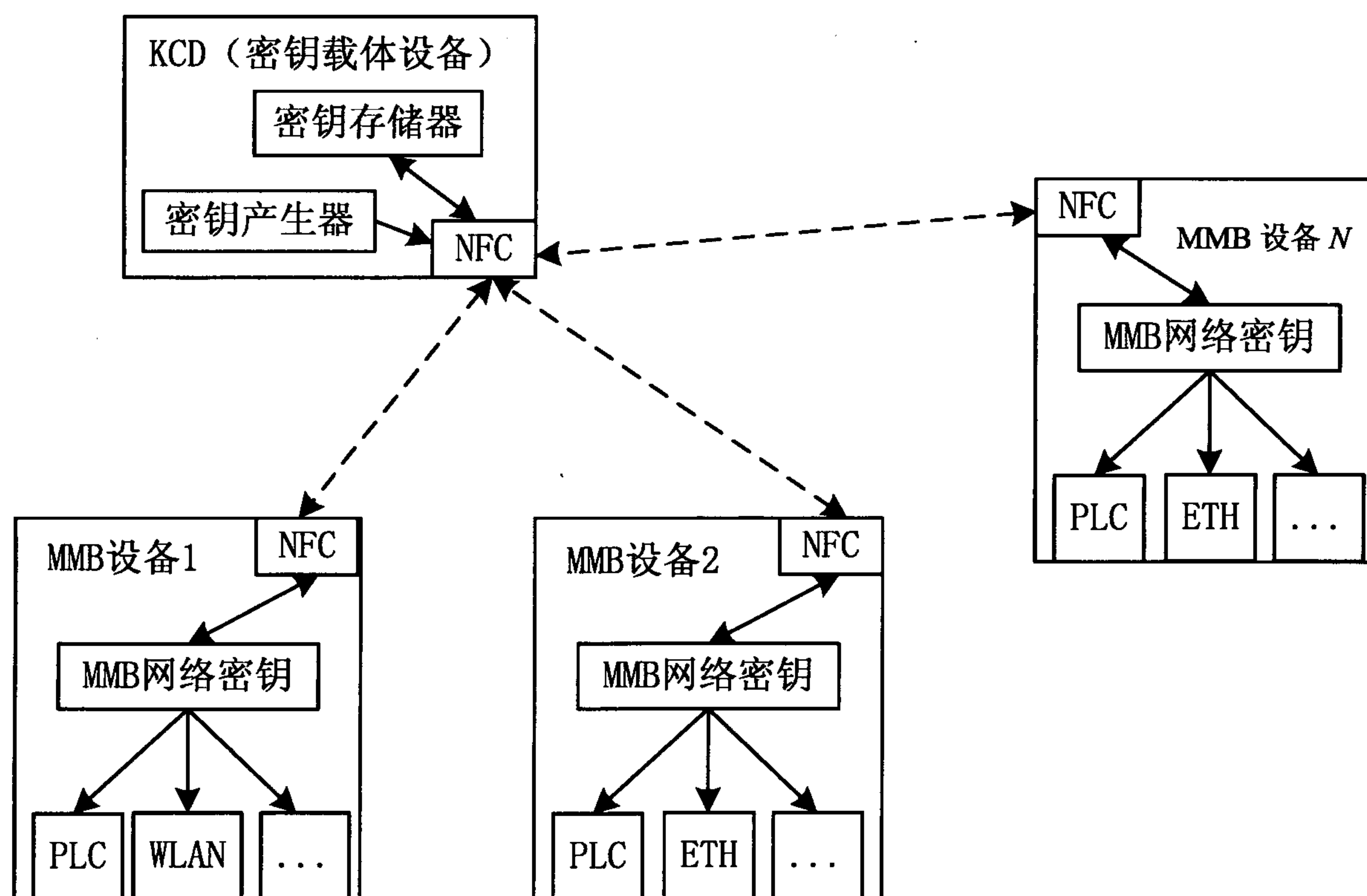
图6 NFCNK 配置过程
