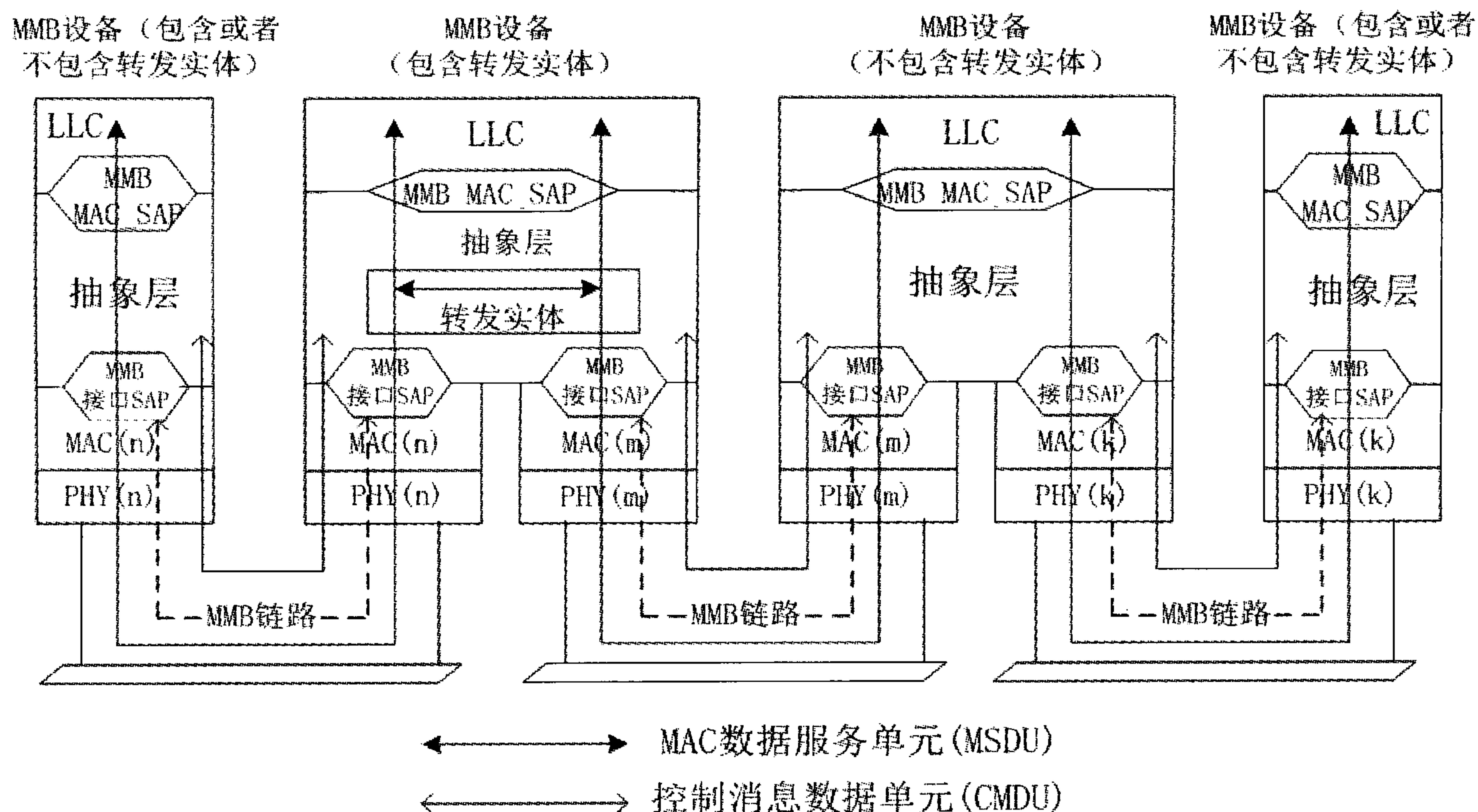
图2 MMB 宽带客户网络设备的互连方式
