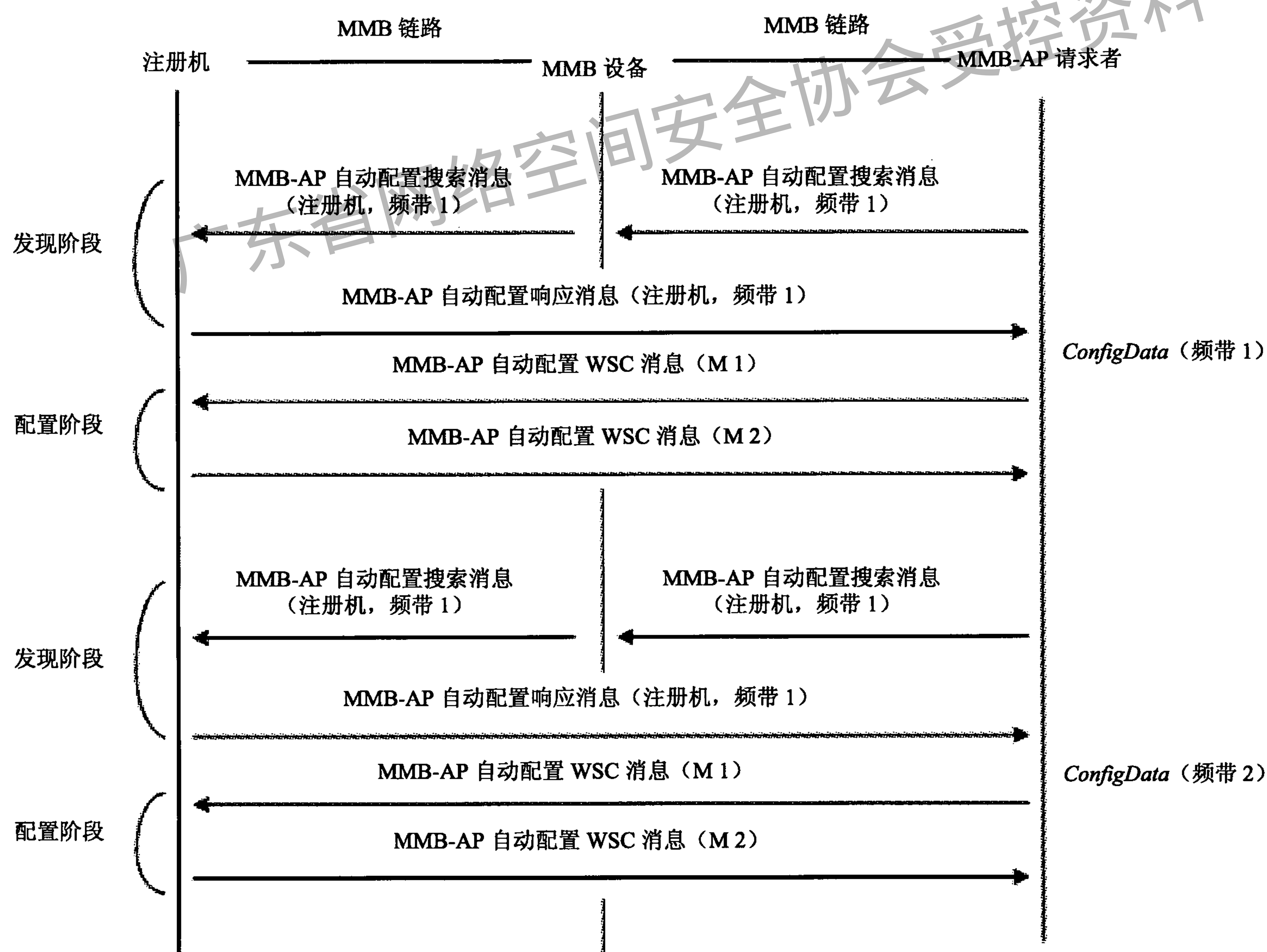
图9 注册机发现过程
