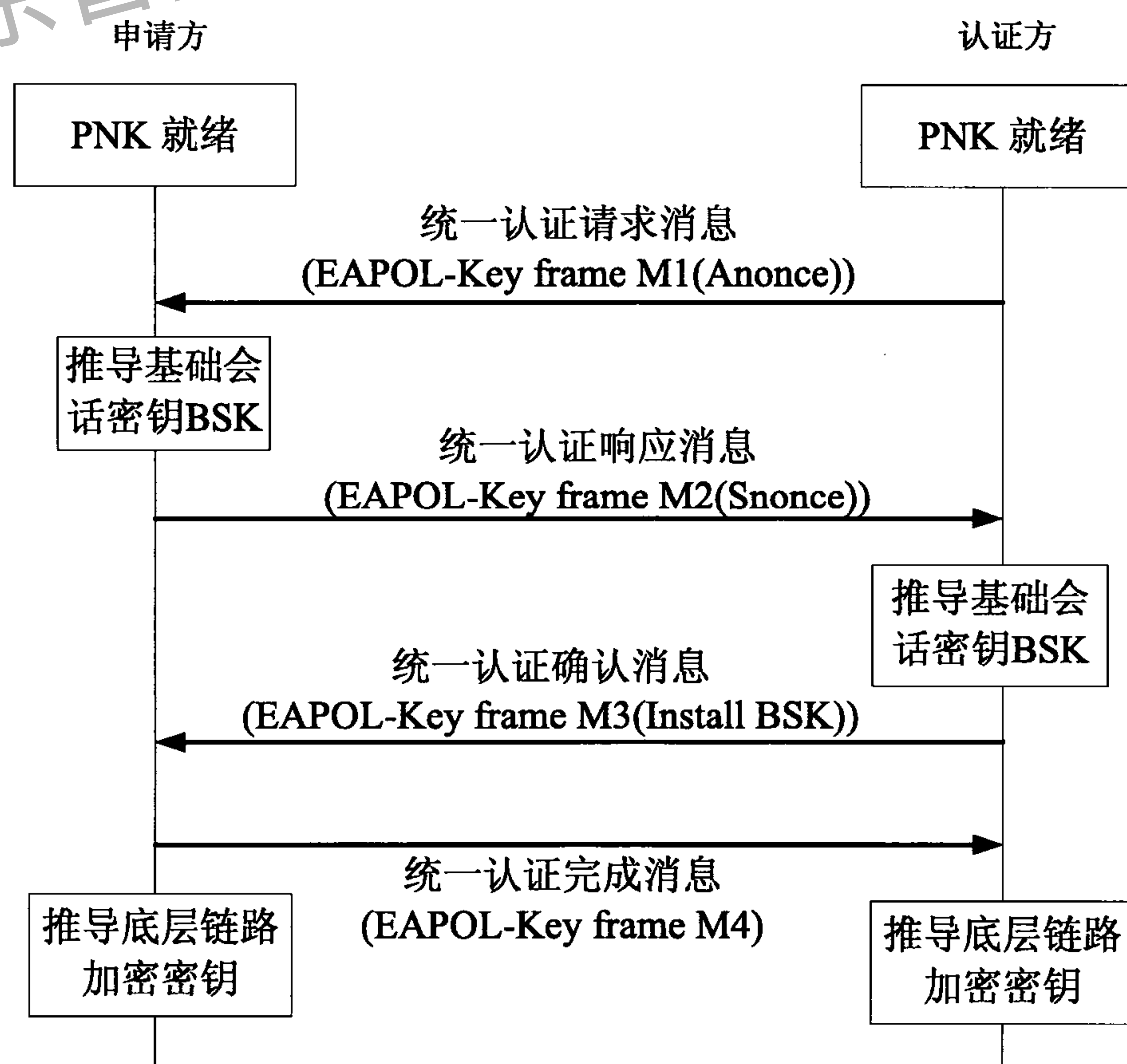
图7 抽象层认证和密钥协商
