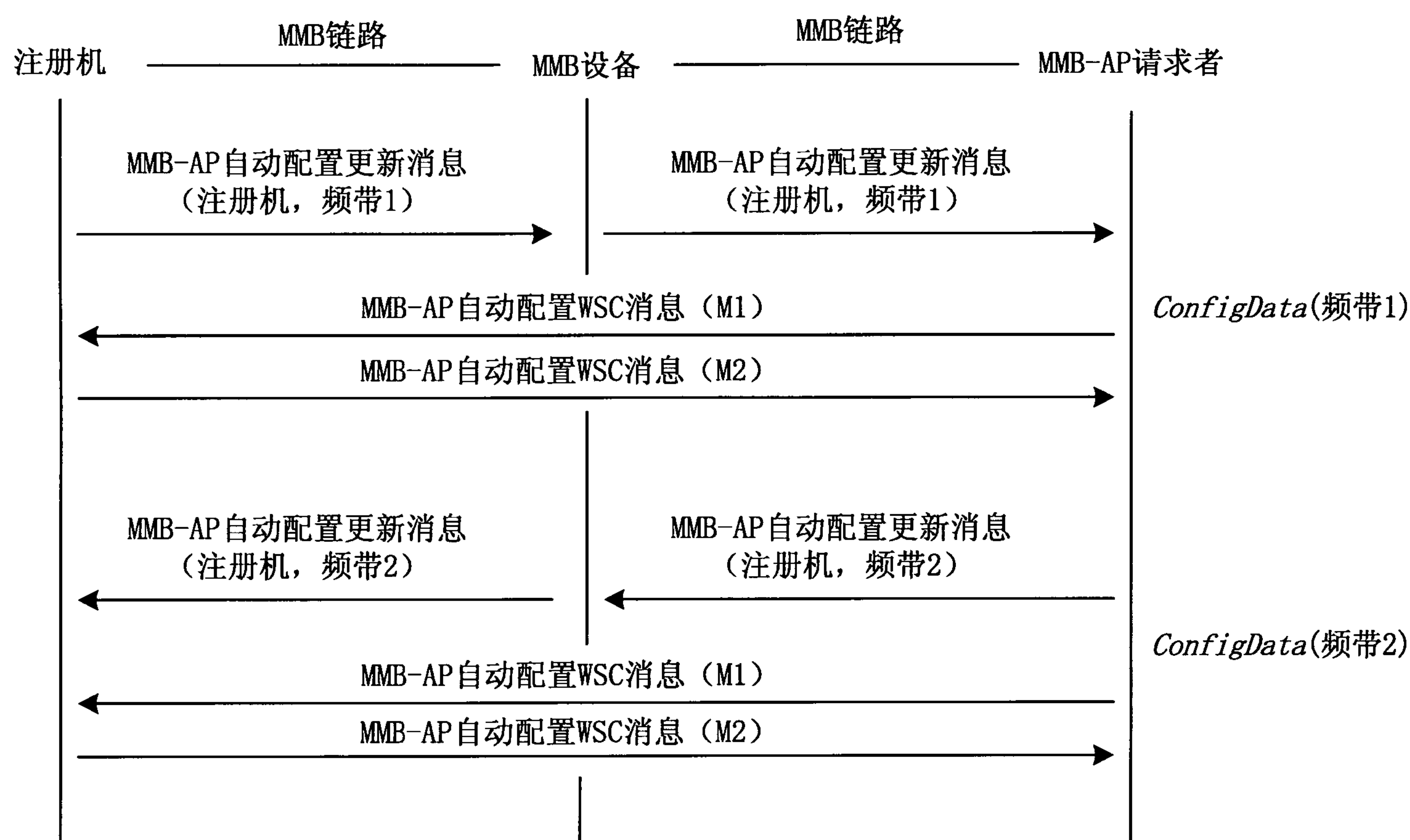
图10 配置更新过程
