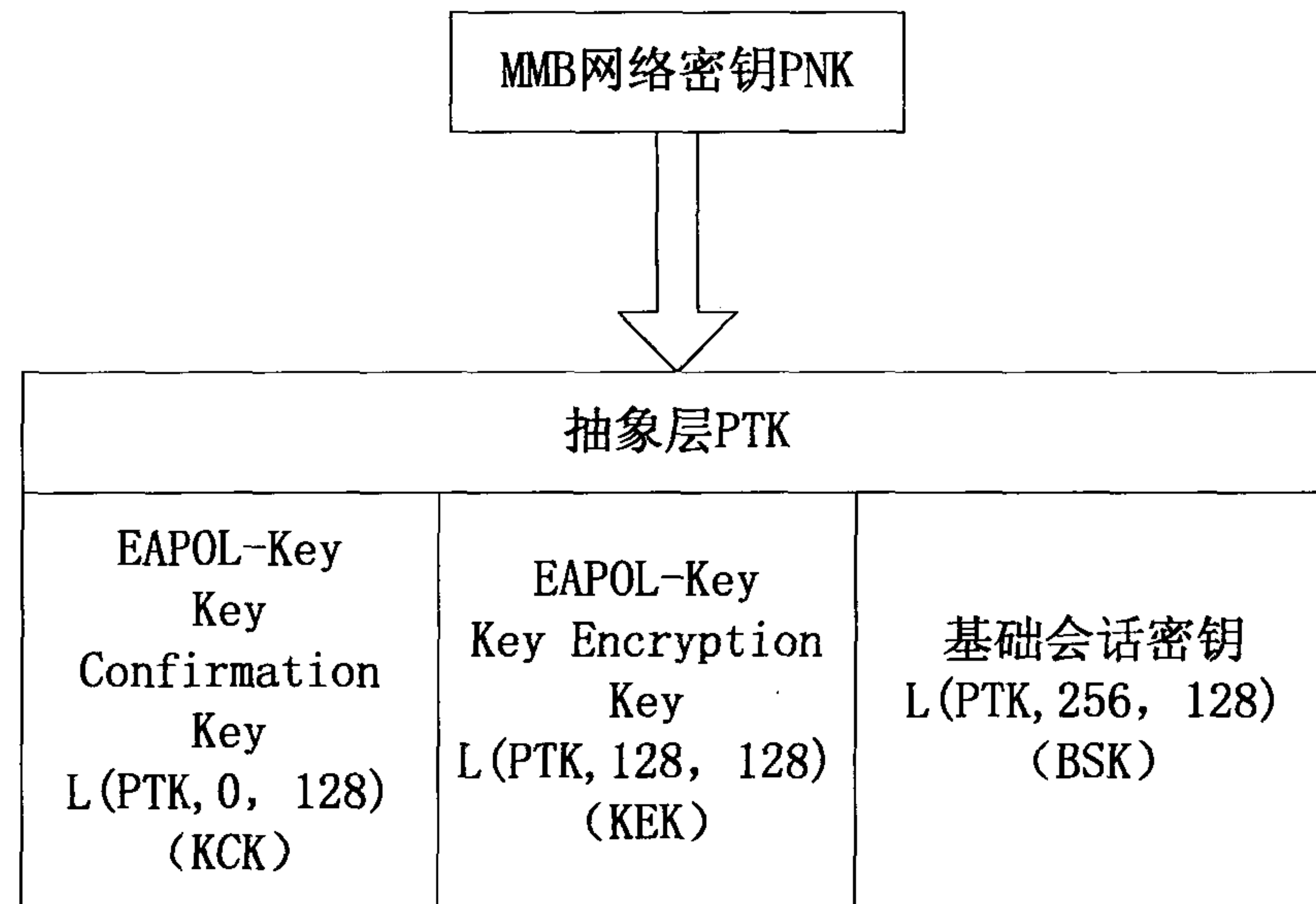
图8 MMB 网络密钥 PNK 推导抽象层 PTK
