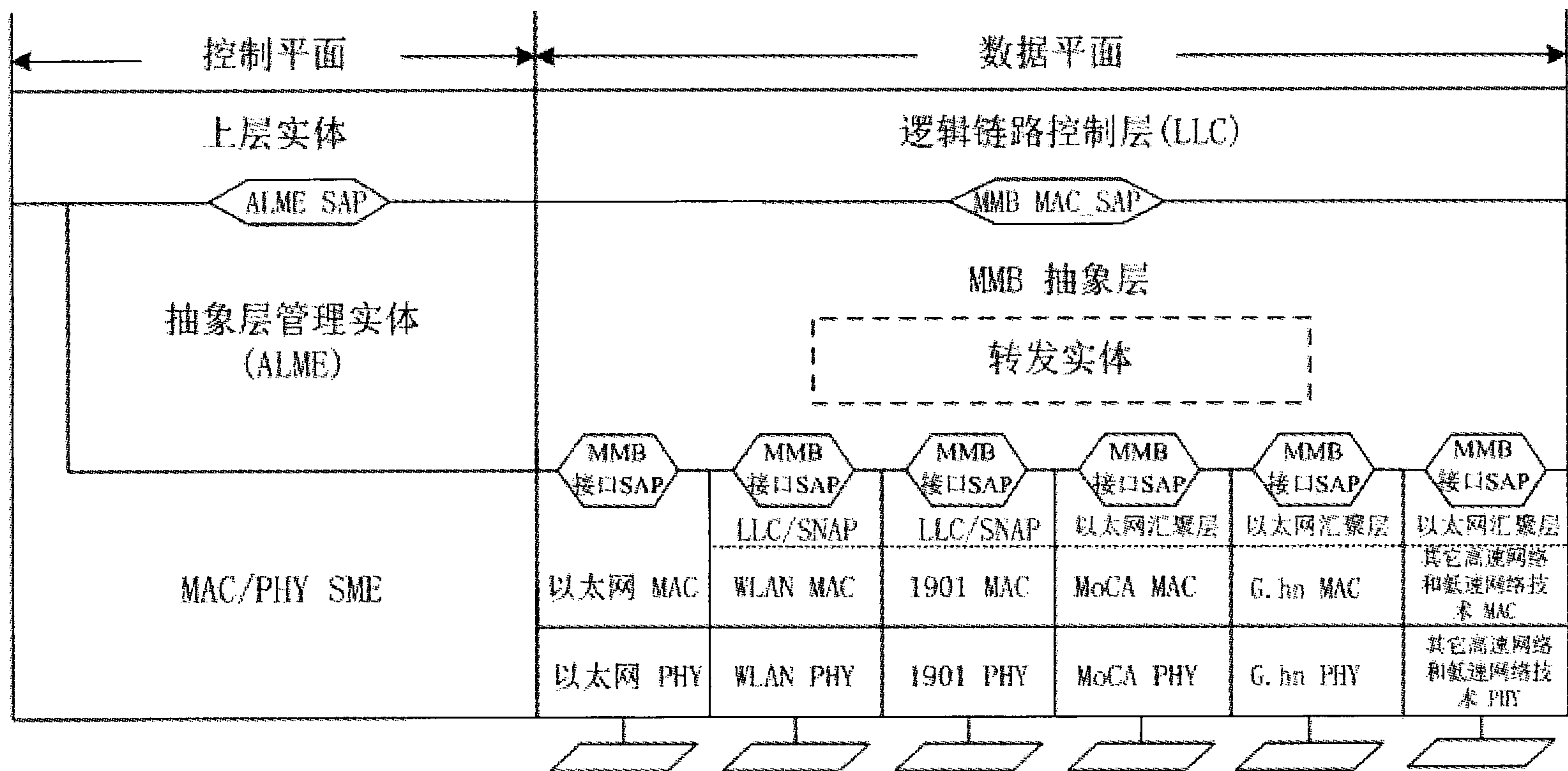
图1 MMB 宽带客户网络的参考模型
