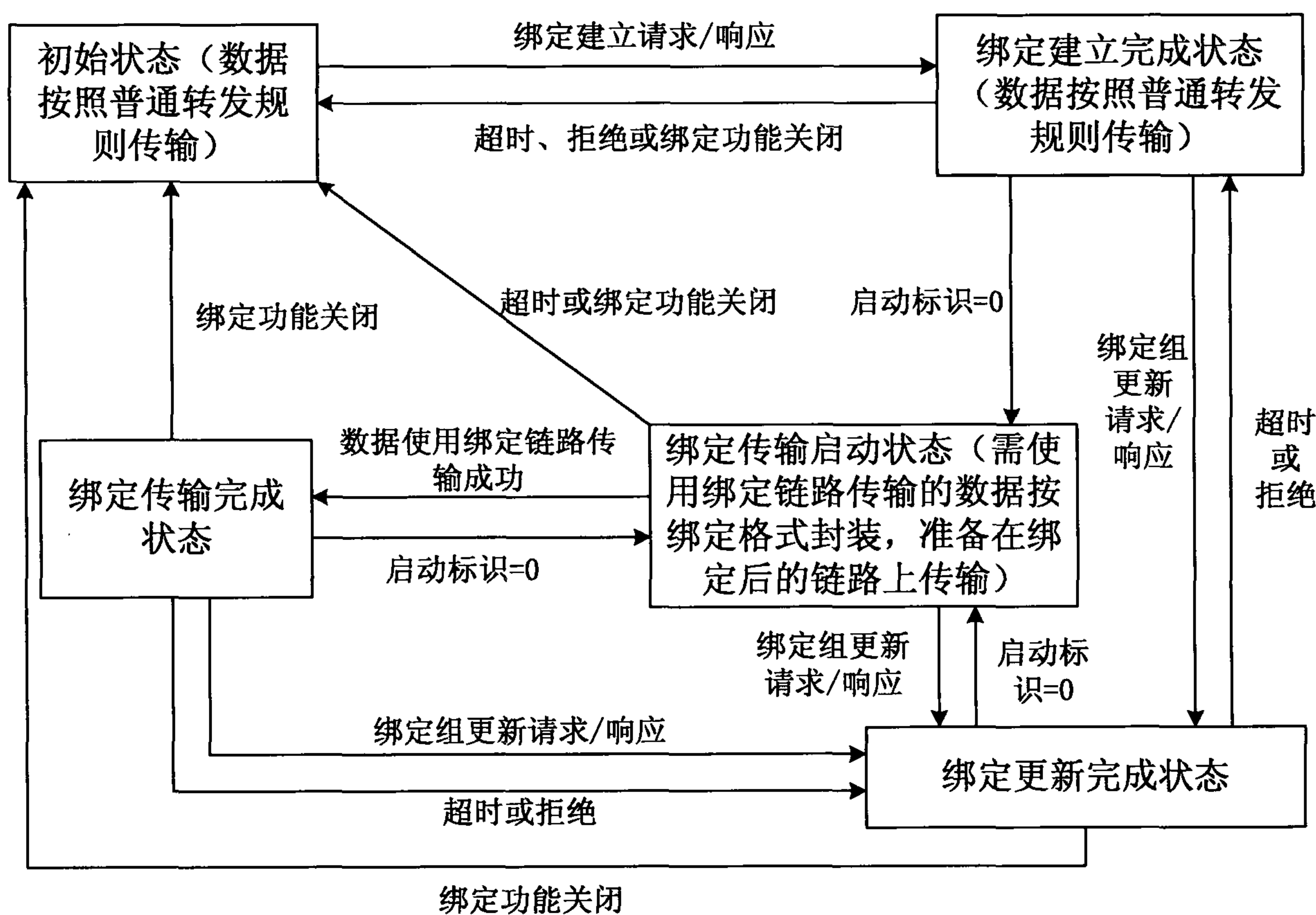
图12 多介质链路绑定的功能状态机
