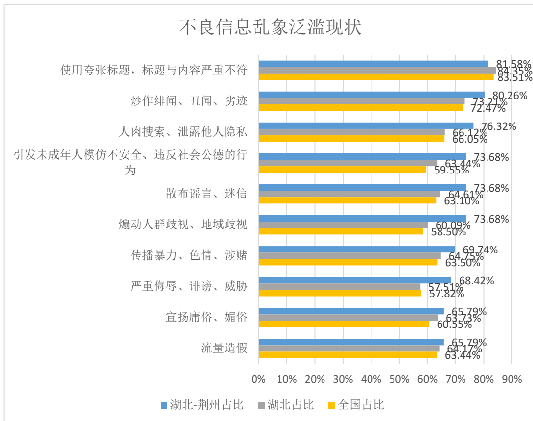
图表 44：不良信息乱象泛滥现状
