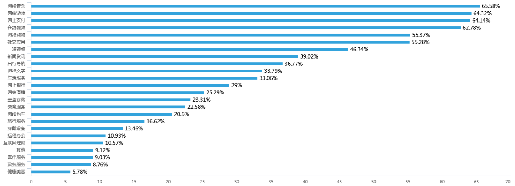
图：常用应用
