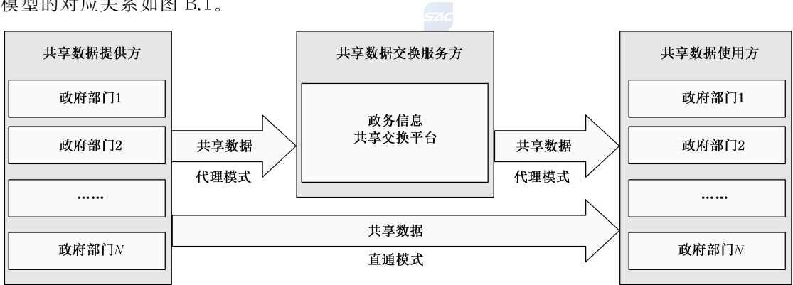
图 B.1 政务信息共享交换代理模式与直通模式
